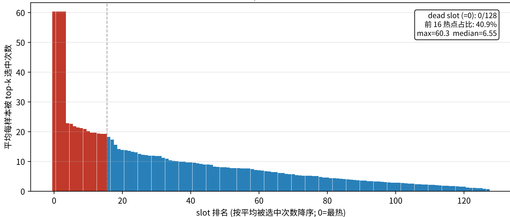
128-slot 路由调用分布 | qa5 32k, n=40, top_k=16/128
