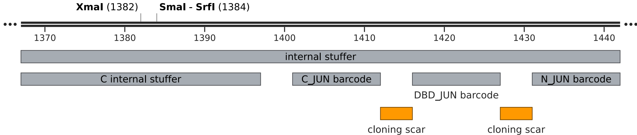
AP-1 DESynR round 3 1368 .. 1442 (75 bp)
