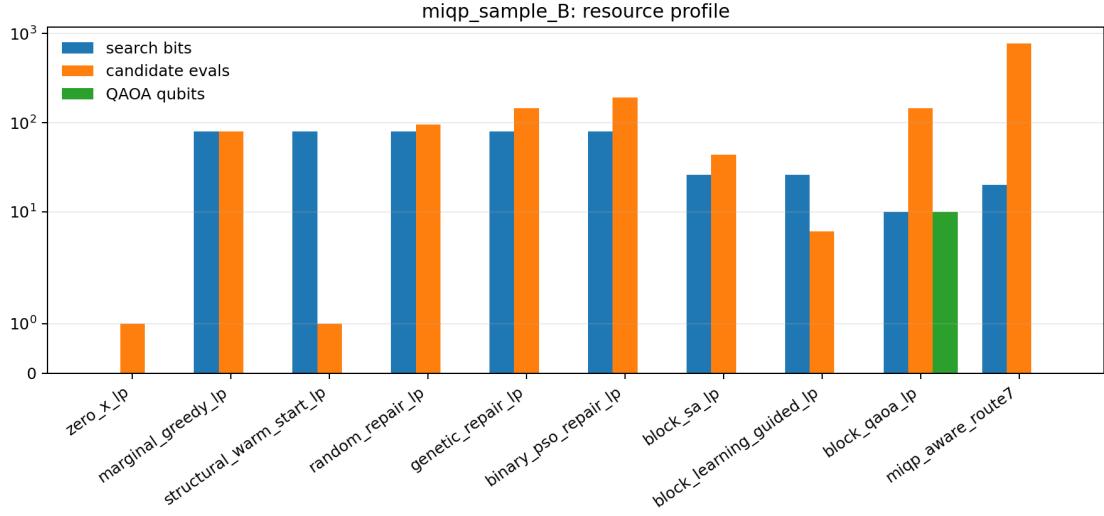
图 6: 样例 B 资源画像。全局精确枚举和全局二进制 QUBO 在 n = 80 时被标注跳过; block-QAOA 控制在 10 qubit, 而 proposed route7++ 使用 20-bit block 和 768 次候选评估达到官方最优。
