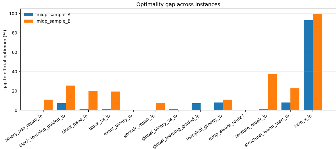
图 3: 跨样例最优性 gap 对比。样例 A 中 proposed route7 与精确枚举同为 0% gap；样例 B 中 proposed route7++ 达到 0% gap，显著优于贪心、随机修复、GA/PSO、block SA、learning-guided 与 block-QAOA 单步候选。
