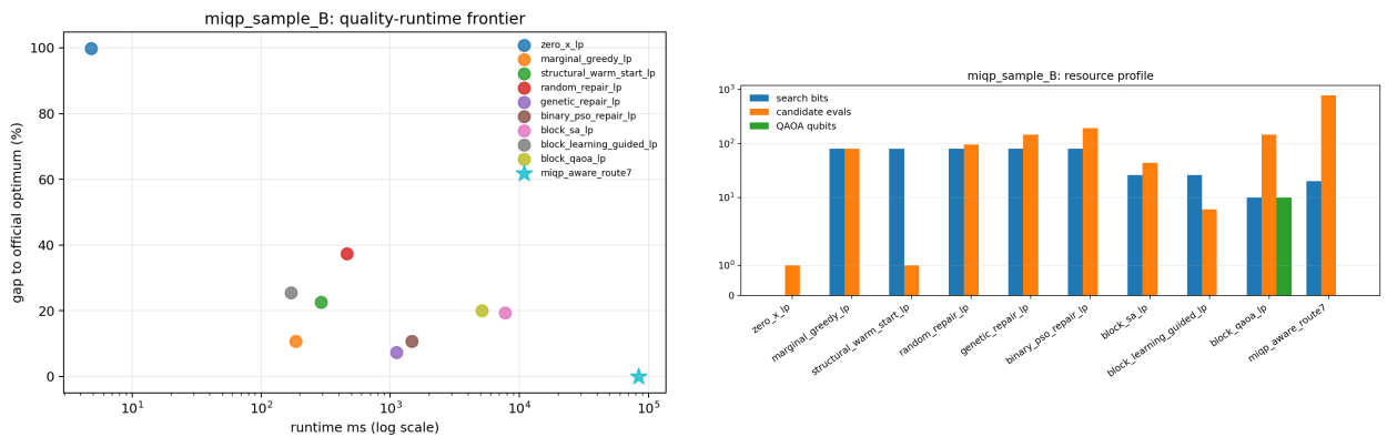
图 4: 左: 样例 B 的质量-时间前沿，QBB-MIQP 用更多 LP 评估换取 0% gap。右: 样例 B 资源画像，block-QAOA 控制在 10 qubit，QBB-MIQP 使用 20-bit block 和 768 次候选评估达到官方最优。
