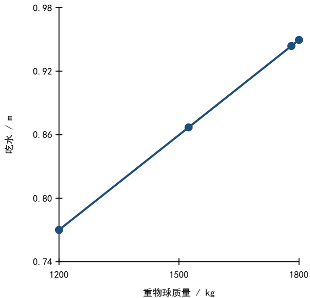
(a) 配重与浮标吃水
