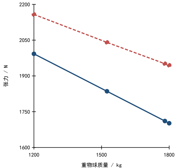
(b) 锚链顶端张力
