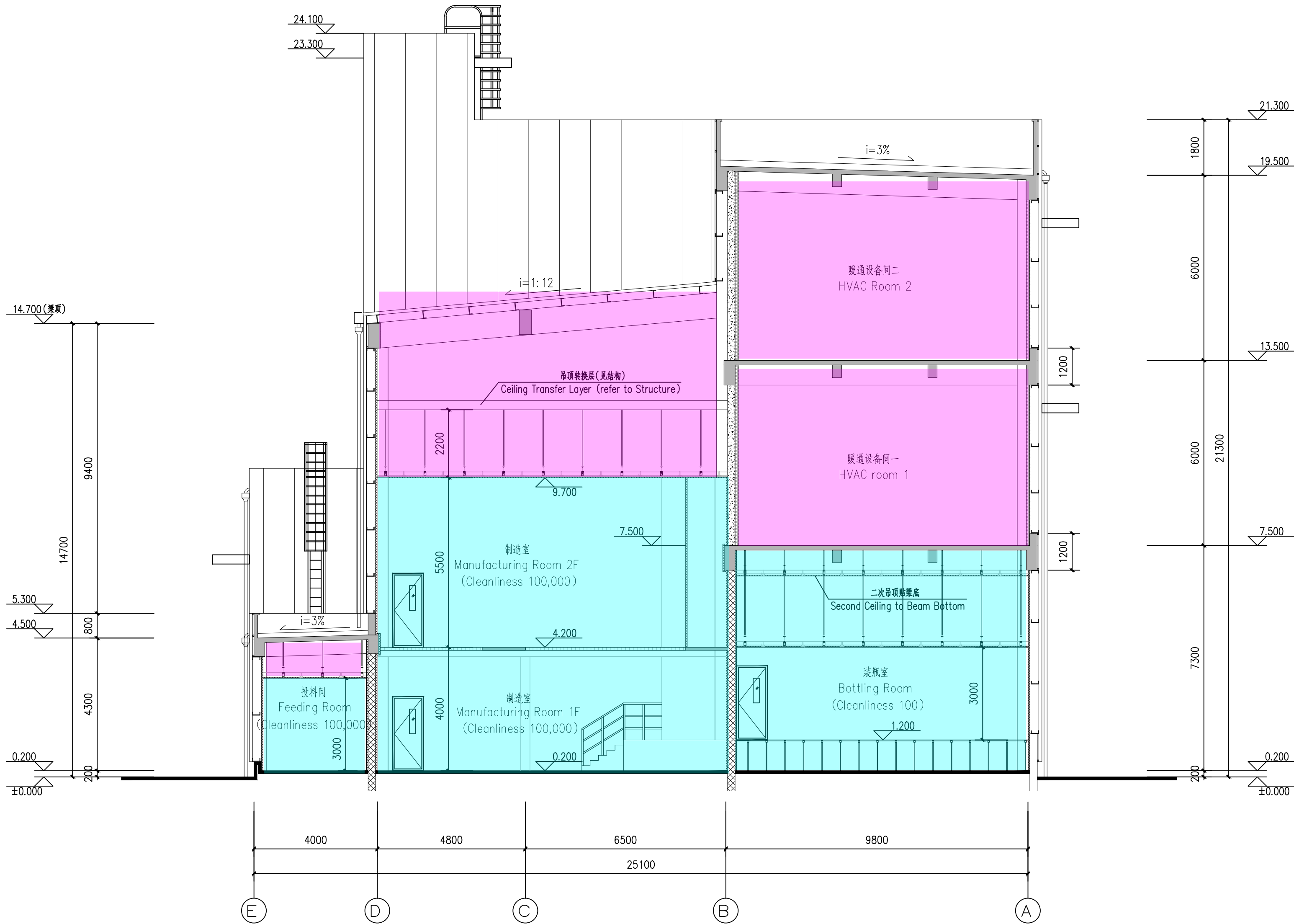
1-1 剖面图 1-1 Section 1:100
