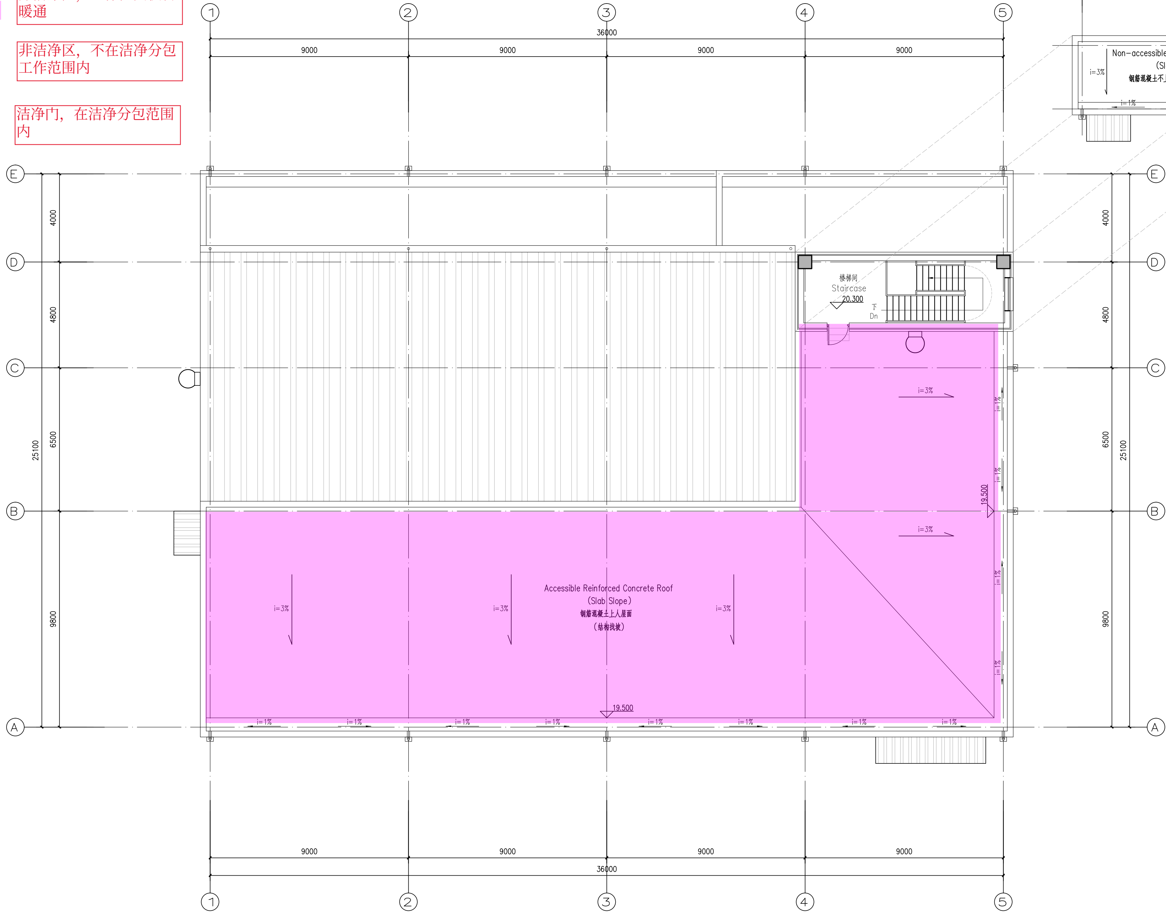
屋顶平面图 Roof Plan 1: 100
