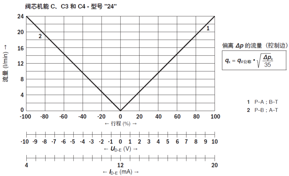
图 0.1 元件样本：流量特性 "L"
