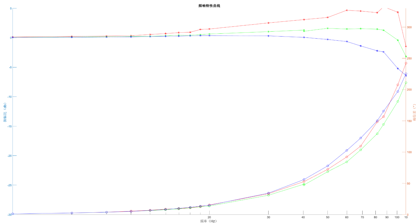
图 12 阀芯频率响应特性曲线
