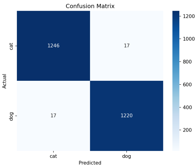
图 7: SE-ResNet34 验证集混淆矩阵
