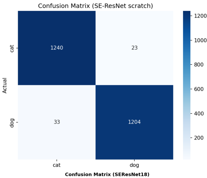
图 7: SE-ResNet18 验证集混淆矩阵
