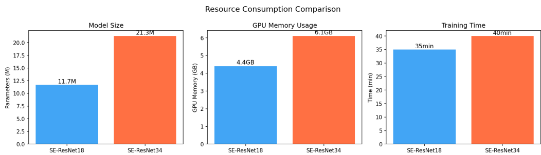
图 10: 资源消耗对比 (参数量、显存、训练时间)
