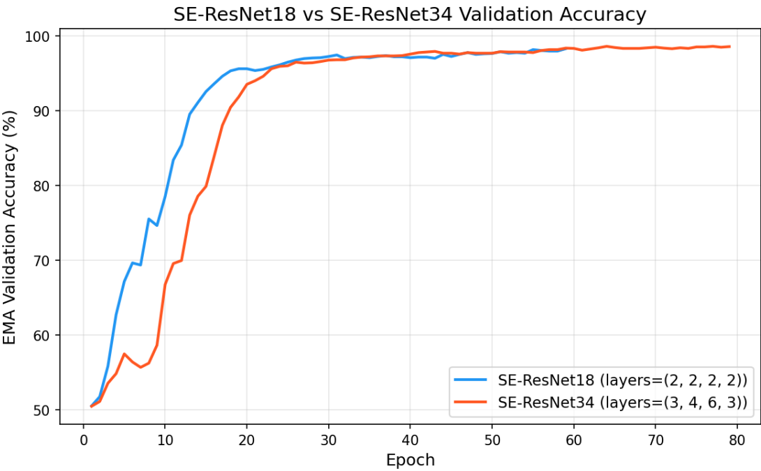
图 3: SE-ResNet18 与 SE-ResNet34 验证精度对比曲线
