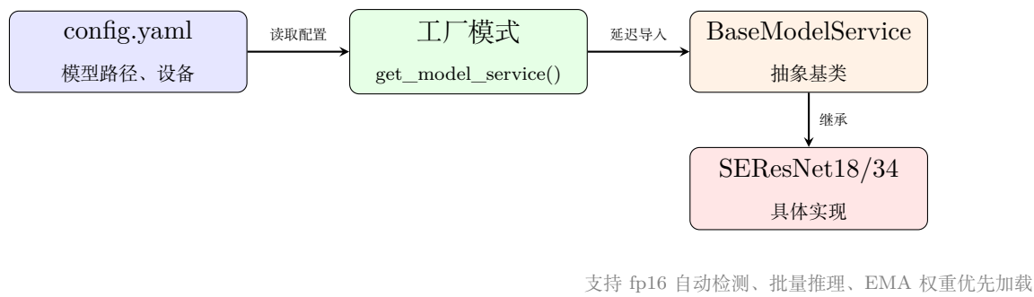
图 11: 模型服务部署架构
