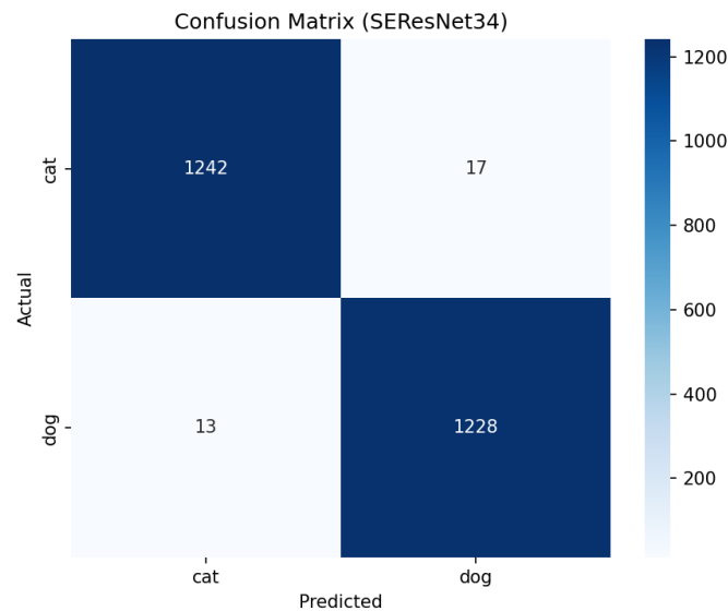
图 8: SE-ResNet34 验证集混淆矩阵
