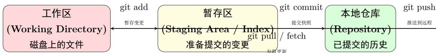
图 1.3: Git 三大工作区域与远程仓库——工作区、暂存区、本地仓库、远程仓库之间的数据流转
