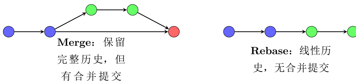
图 4.5: Merge 与 Rebase 的对比——Merge 保留完整历史产生合并节点，Rebase 生成线性历史
