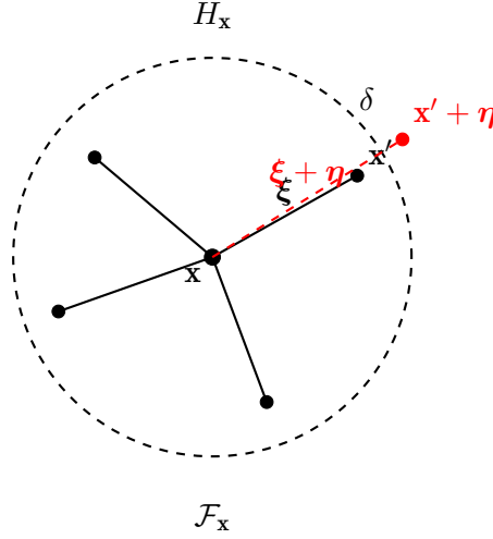
图 2.5 物质点、键、近场域与族的整合示意，族 \mathcal{F}_x 为近场域 H_x 内与 x 通过键相连的物质点集合
