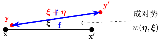
图 2.7 微弹性材料中，成对势 w 在键两端对称，导出的对力 \mathbf{f} 沿变形后键方向并满足反作用条件
