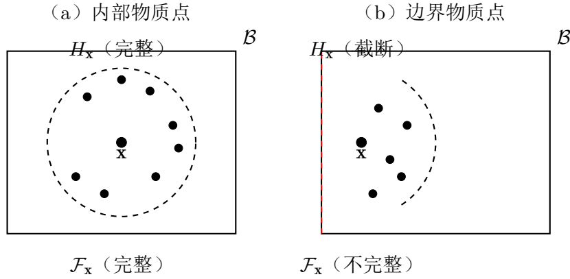
图 2.4 内部物质点与边界物质点的近场域和族对比: 边界附近的物质点其近场域被物体边界截断, 族不完整, 导致表面效应 (surface effect, 详见第 10 章) [33, 41]
