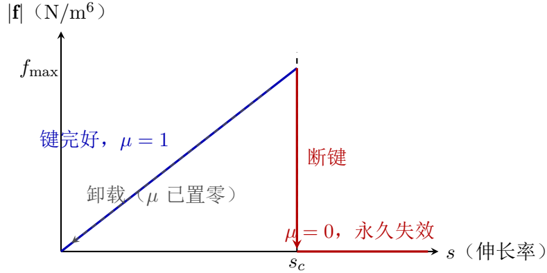
图 2.9 对力函数 |\mathbf{f}| 与伸长率 s 的关系示意：加载阶段键伸长， |\mathbf{f}| 按本构关系增长；当 s 首次达到 s_c 时键断裂， |\mathbf{f}| 骤降为零；此后该键永久失效，卸载路径沿原本构曲线返回原点但历史变量 \mu 已置零
