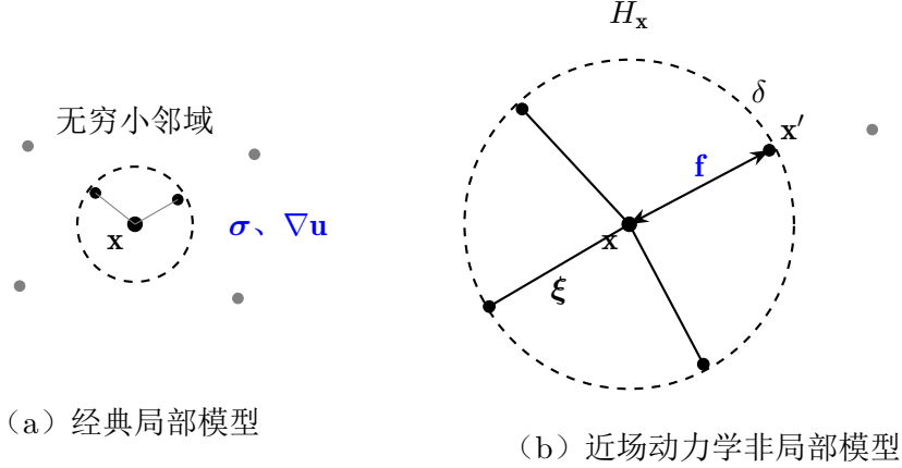
图 2.1 经典局部连续介质力学与近场动力学在物质点相互作用方式上的对比，左图为经典局部模型，其力学状态由该点处的应力张量 \sigma 与变形梯度 \nabla \mathbf{u} 完全决定，右图为近场动力学非局部模型，物质点通过键与近场域 H_x （半径 \delta ）内的远处物质点直接相互作用
