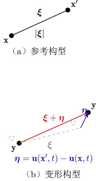
图 2.2 键的几何关系：(a) 参考构型；(b) 变形构型
