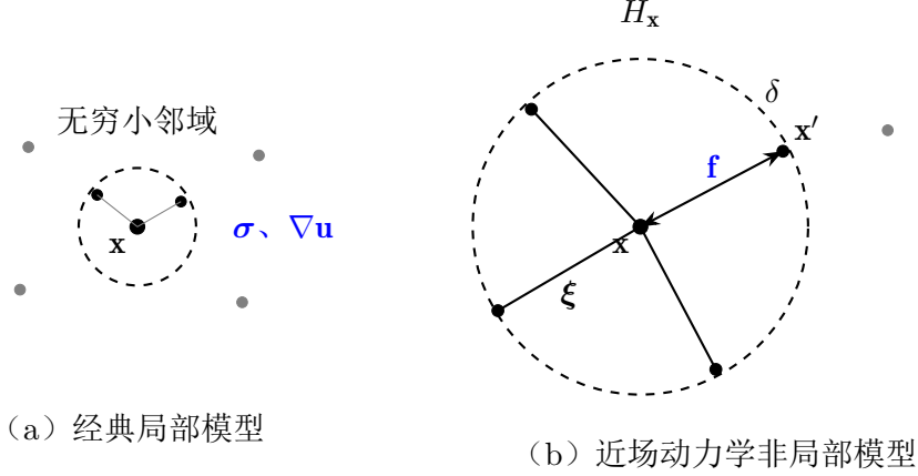
图 2.1 经典局部模型与近场动力学非局部模型的物质点相互作用方式对比
