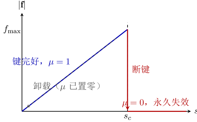
图 2.7 对力函数 |\mathbf{f}| 与伸长率 s 的关系示意: 加载阶段键伸长, |\mathbf{f}| 按本构关系增长; 当 s 首次达到 s_c 时键断裂, |\mathbf{f}| 骤降为零; 此后该键永久失效, 卸载路径沿原本构曲线返回原点但历史变量 \mu 已置零
