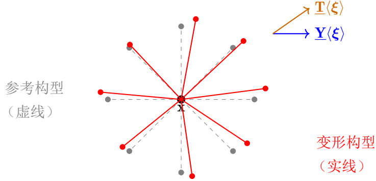
图 2.6 态型理论中，变形态 \underline{Y} 把参考键映射为变形后键，力态 \underline{T} 把参考键映射为力密度矢量。力态依赖整个变形态，而非单条键
