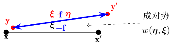
图 2.8 微弹性材料中，成对势 w 在键两端对称，导出的对力 \mathbf{f} 沿变形后键方向并满足反作用条件
