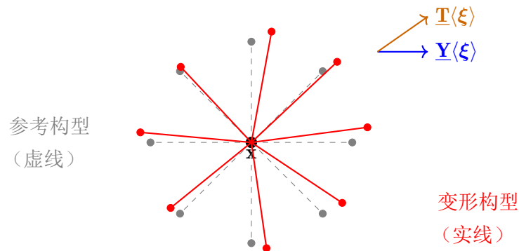
图 2.9 态型理论中, 变形态 \underline{\mathbf{Y}} 把参考键映射为变形后键, 力态 \underline{\mathbf{T}} 把参考键映射为力密度矢量。力态依赖整个变形态, 而非单条键
