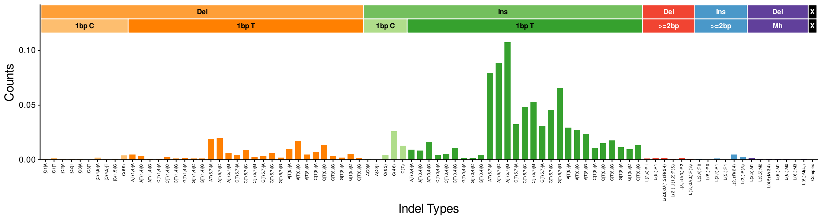
InsDel1c (euclidean: 0.0755)
