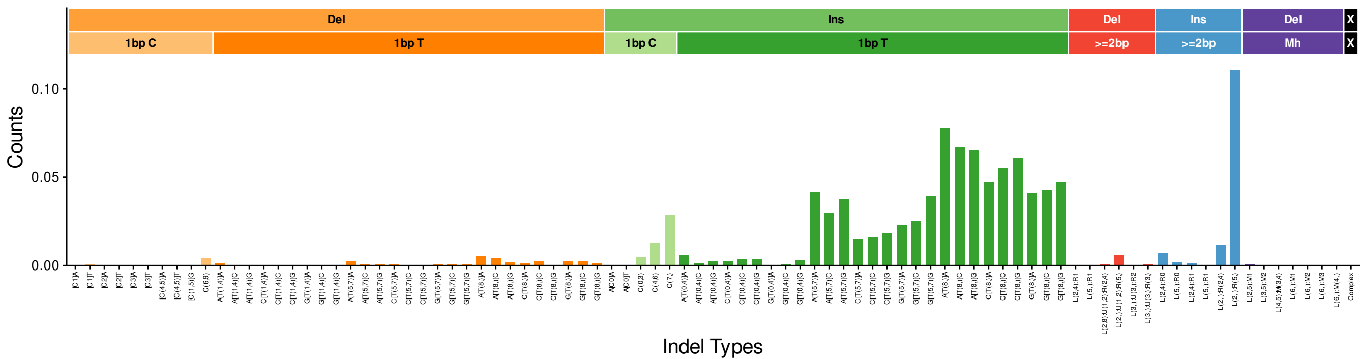
InsDel_O (euclidean: 0.1028)
