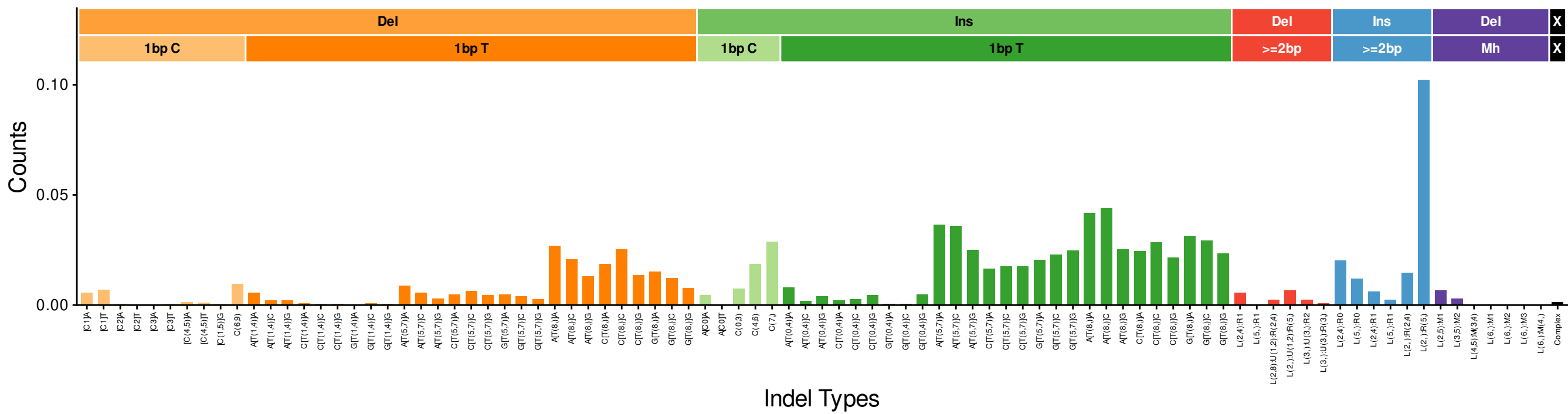
InsDel_O (cosine: 0.8986)
