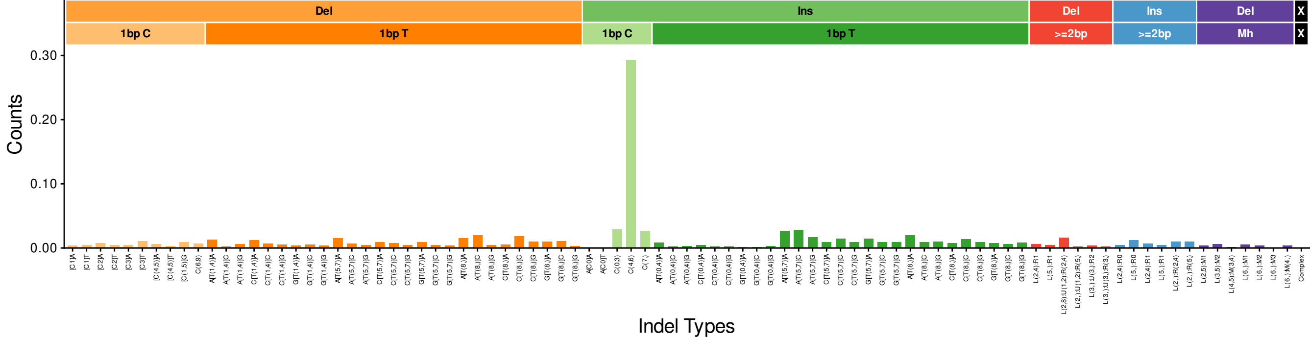
InsDel_L (cosine: 0.9692)
