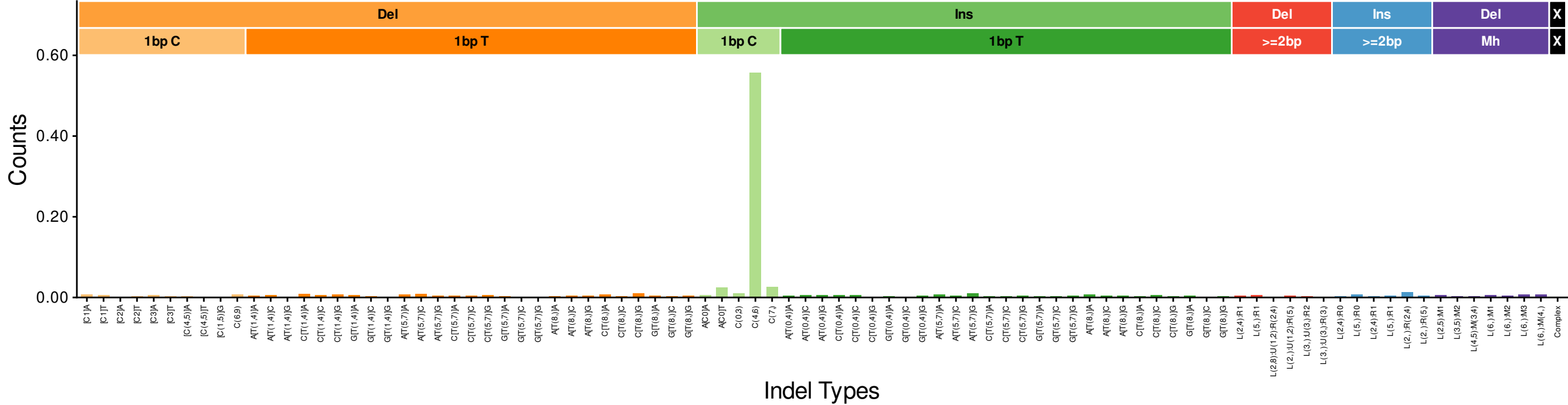
InsDel_L (euclidean: 0.2719)
