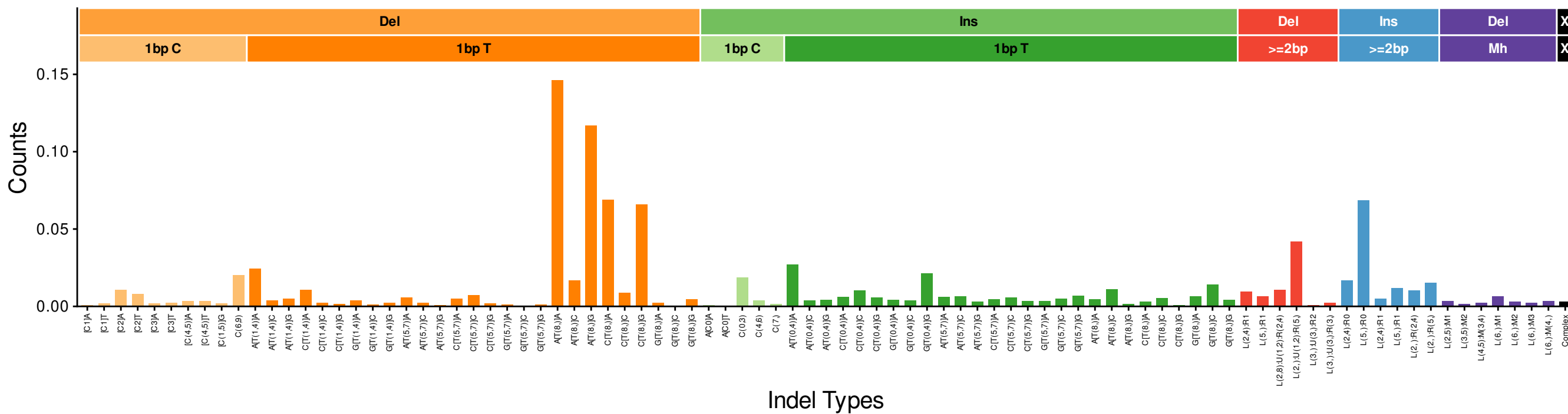
InsDel7 (cosine: 0.7503)
