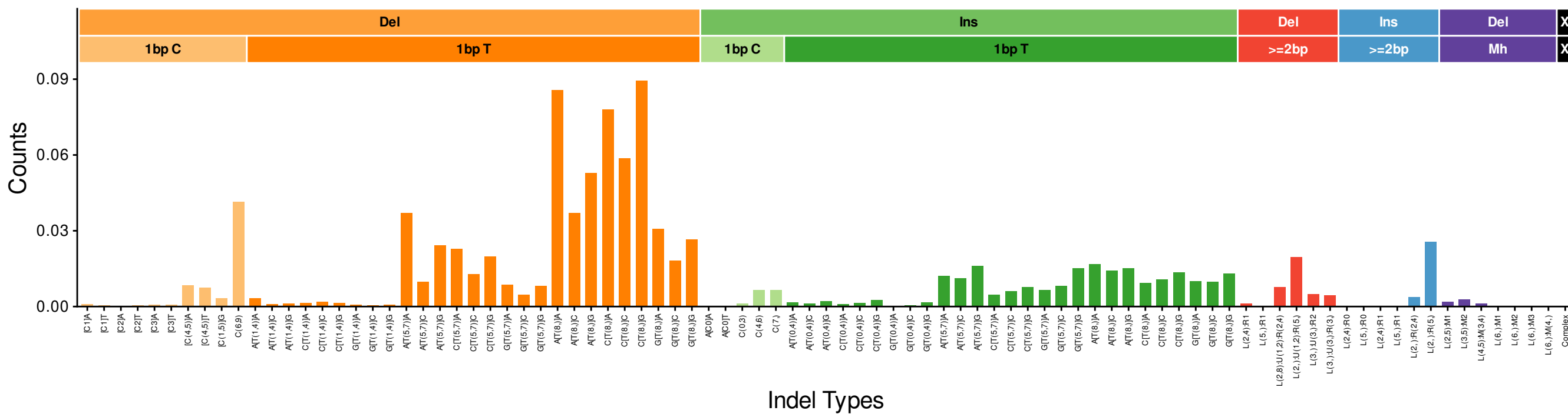
InsDel7 (euclidean: 0.1580)
