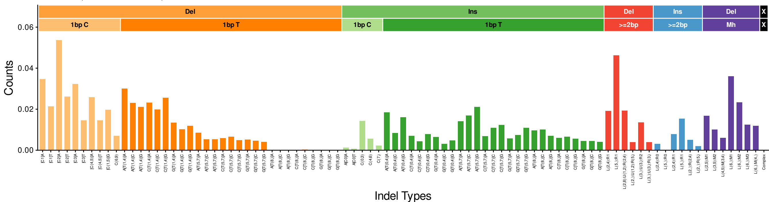
InsDel5b (euclidean: 0.1461)
