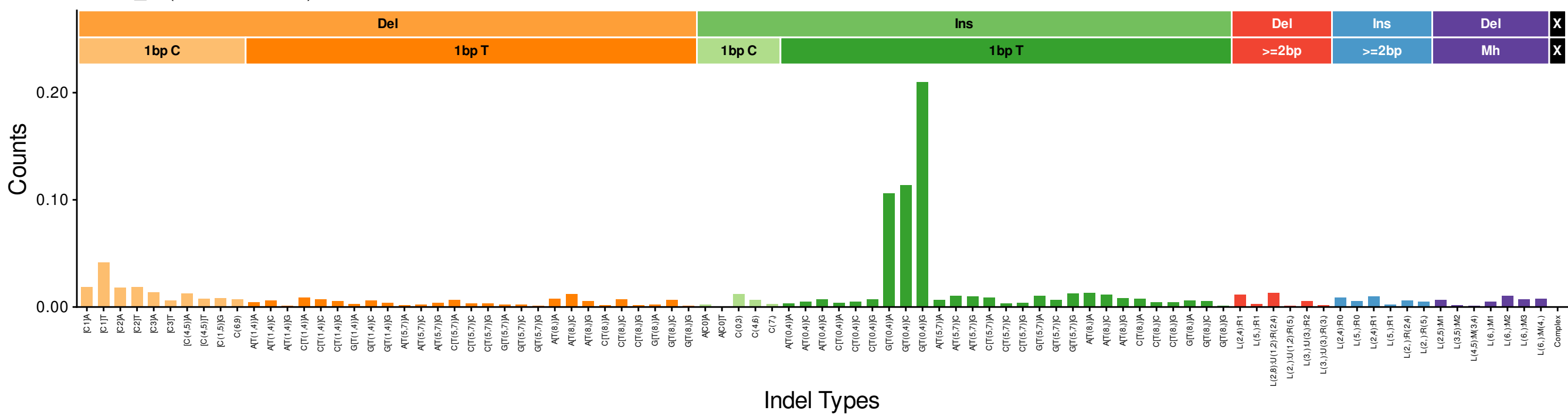
InsDel_G (cosine: 0.8571)
