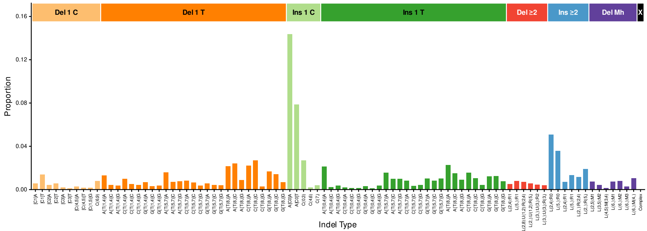
InsDel_D (cosine = 0.898)
