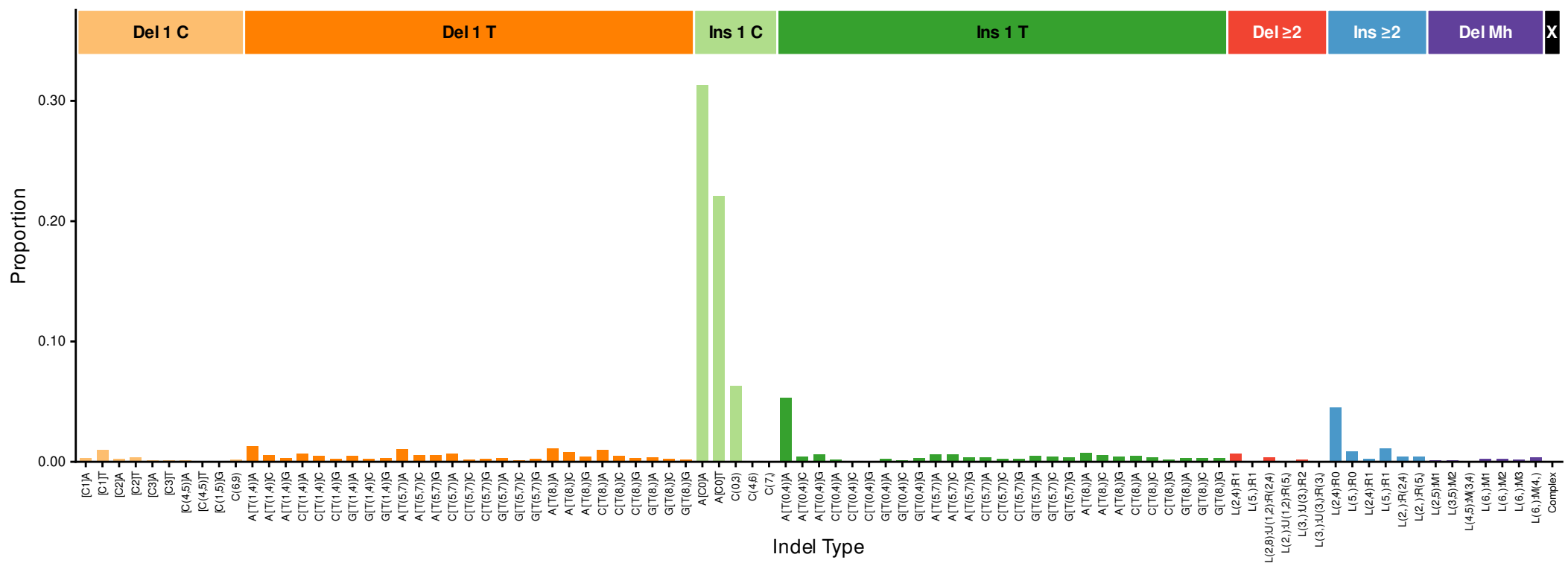
InsDel_D (cosine = 0.898)
