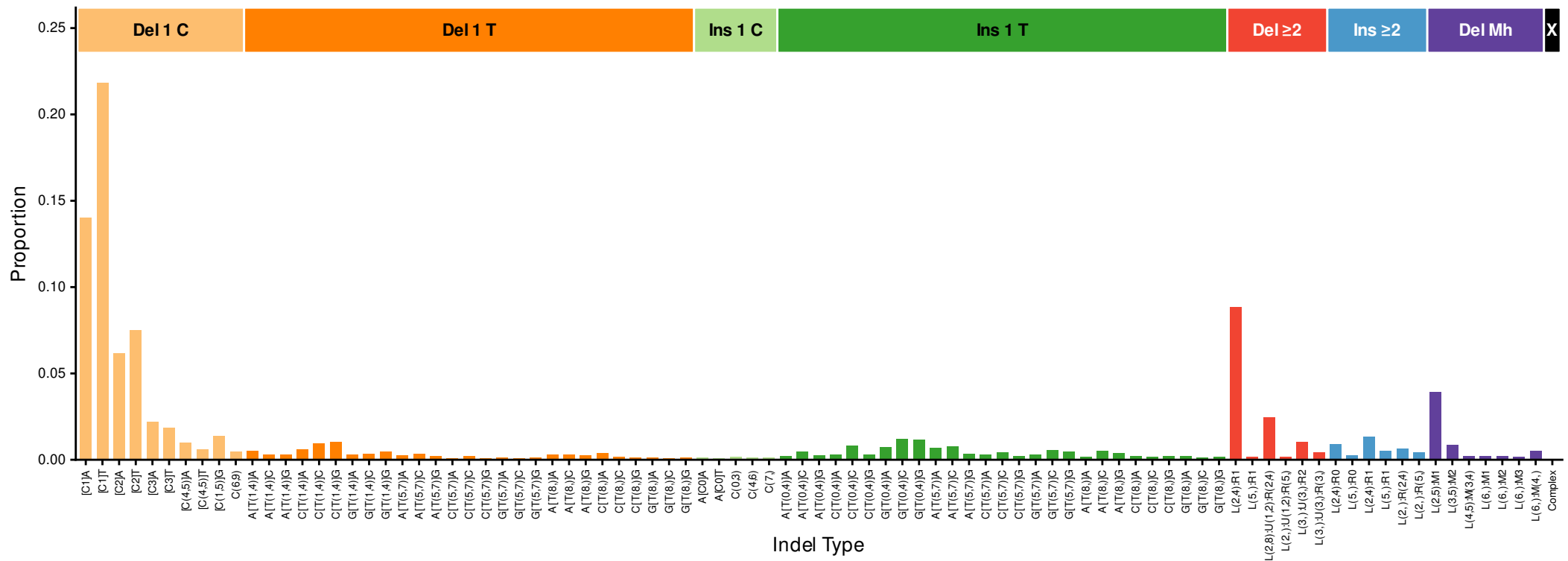
InsDel_A_alpha (cosine = 0.916)
