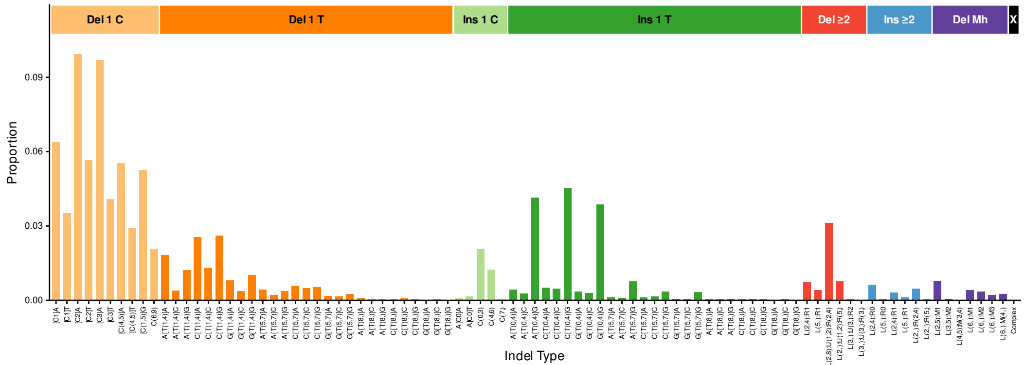
InsDel3a (cosine = 0.907)
