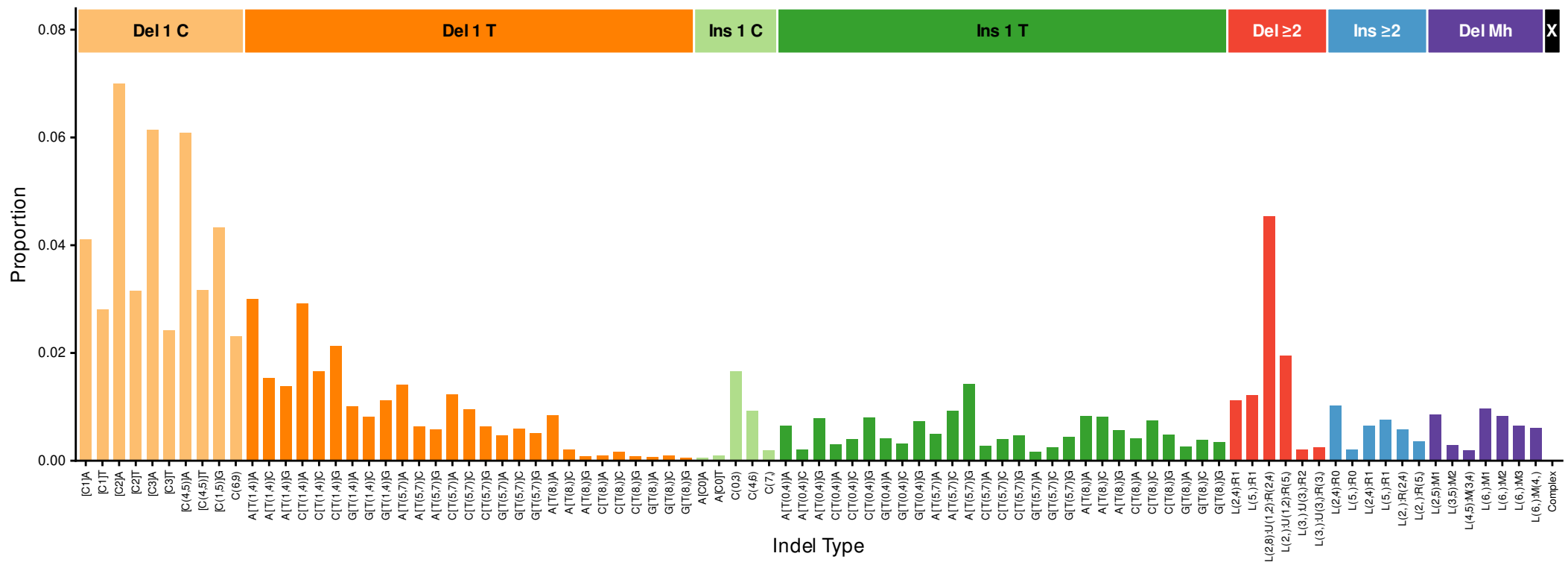
InsDel3a (cosine = 0.907)
