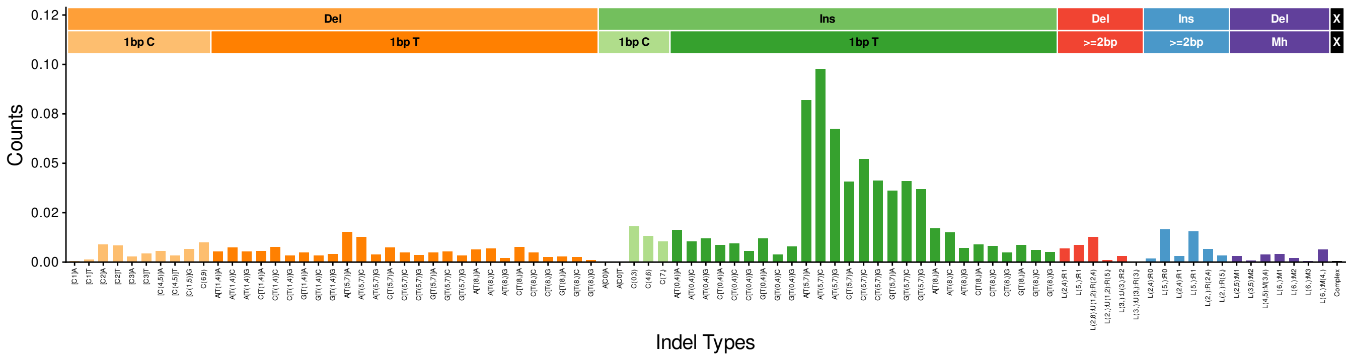
InD14 (euclidean: 0.0753)
