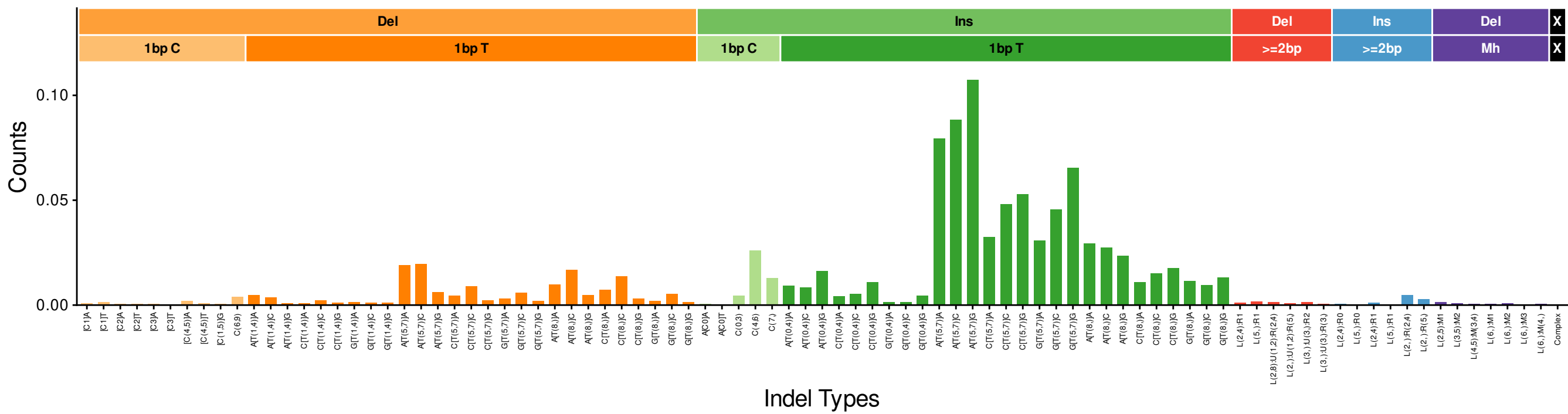
InD11 (cosine: 0.9365)
