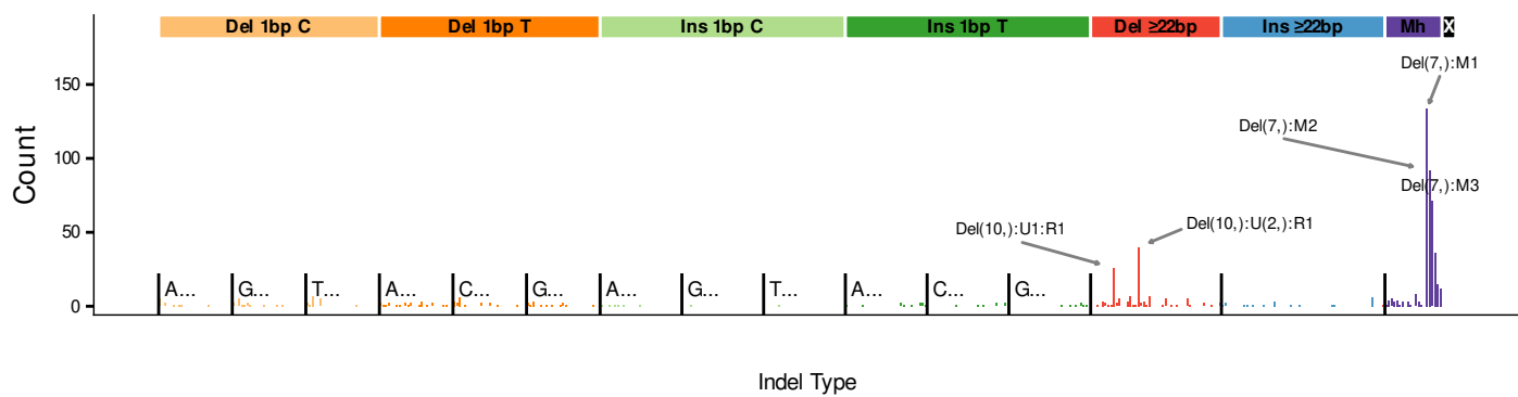
Breast::SP116365 (our type-89 exemplar)
