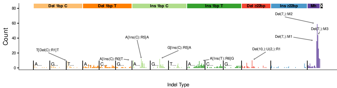
Pancreas::SP70106 (our type-89 exemplar)
