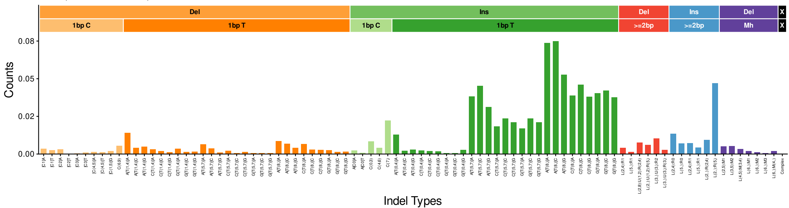
InD1 (euclidean: 0.0363)
