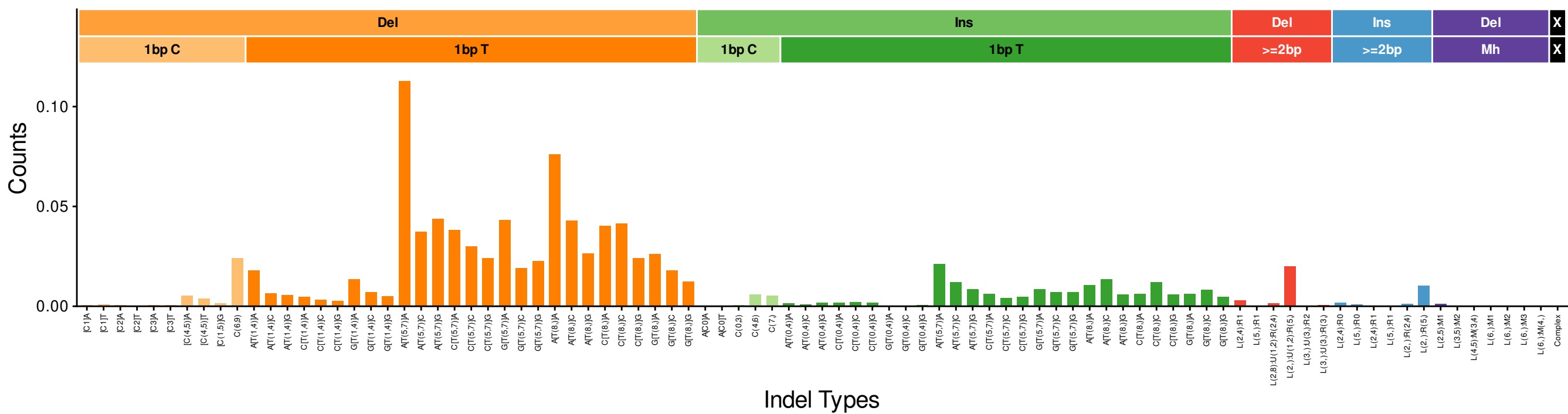
InD16a (euclidean: 0.1438)
