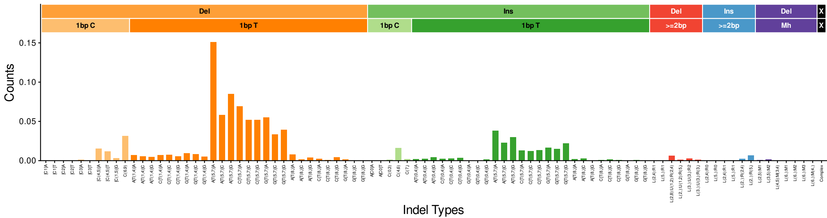
InD16a (cosine: 0.7951)
