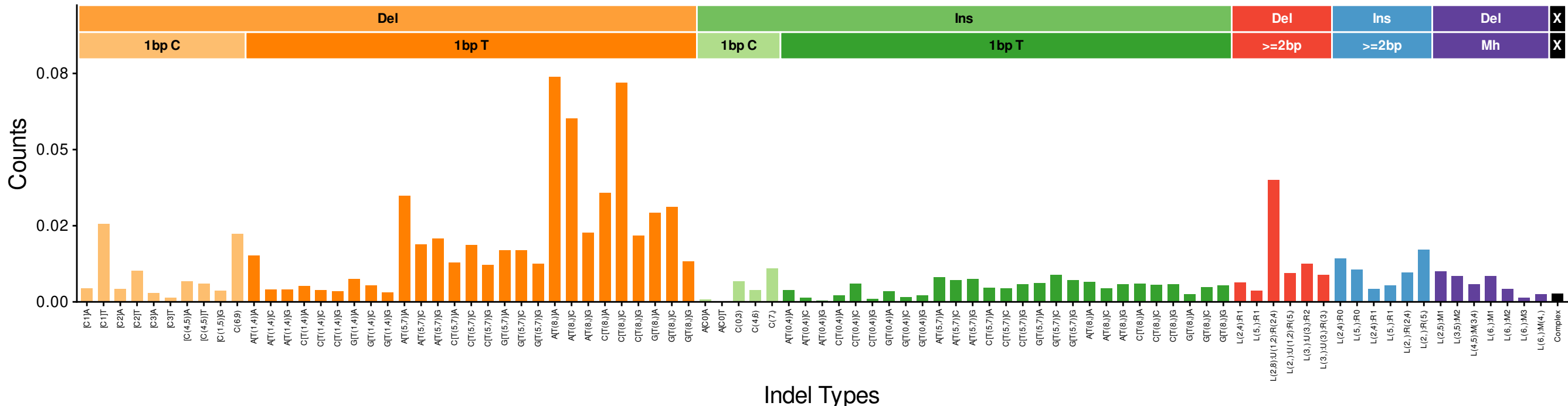
InD2b (euclidean: 0.1435)
