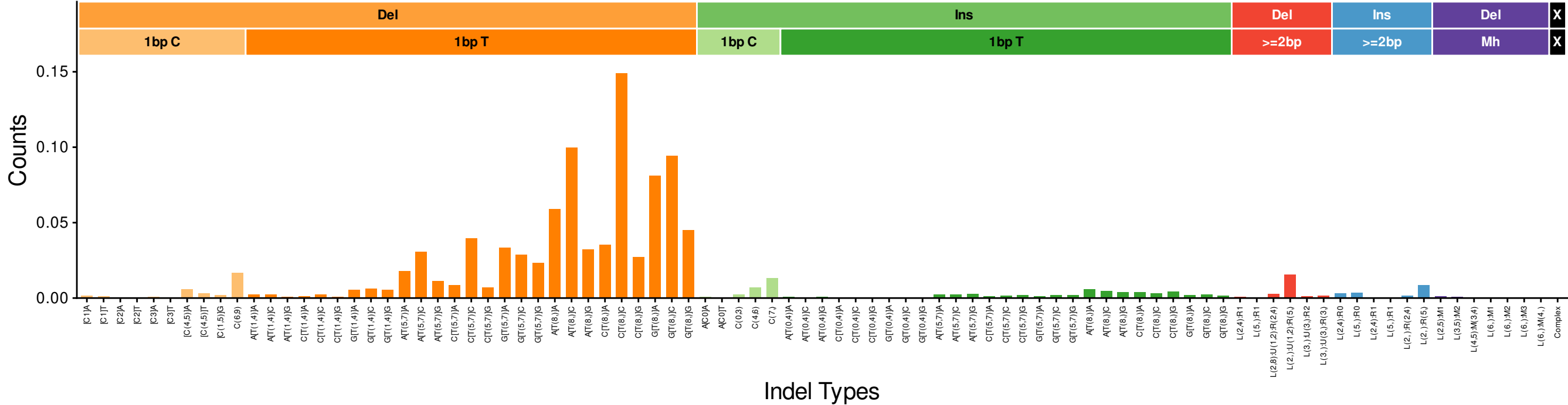
InD2b (cosine: 0.8382)
