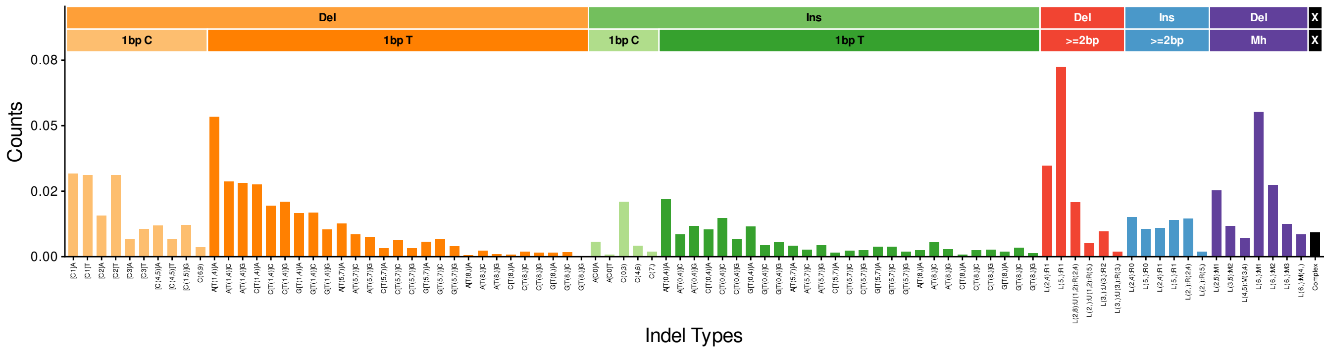
InD29 (euclidean: 0.0587)
