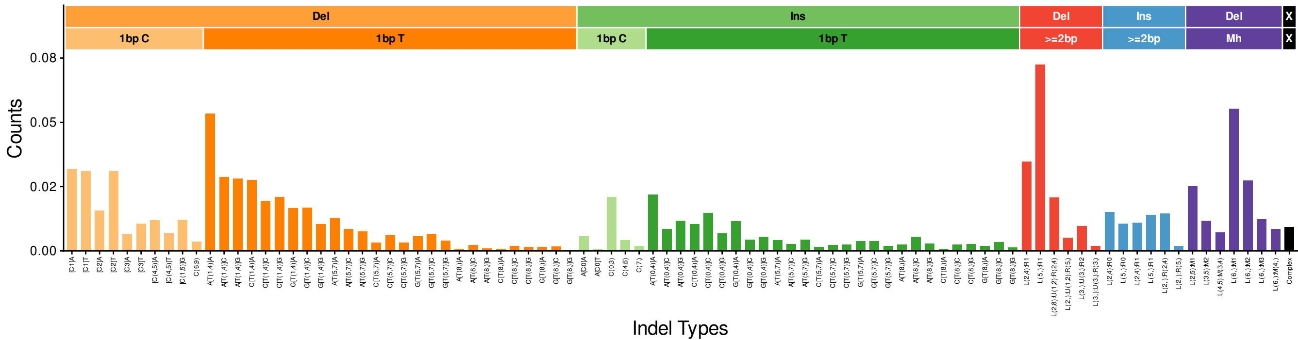
InD29 (euclidean: 0.0587)
