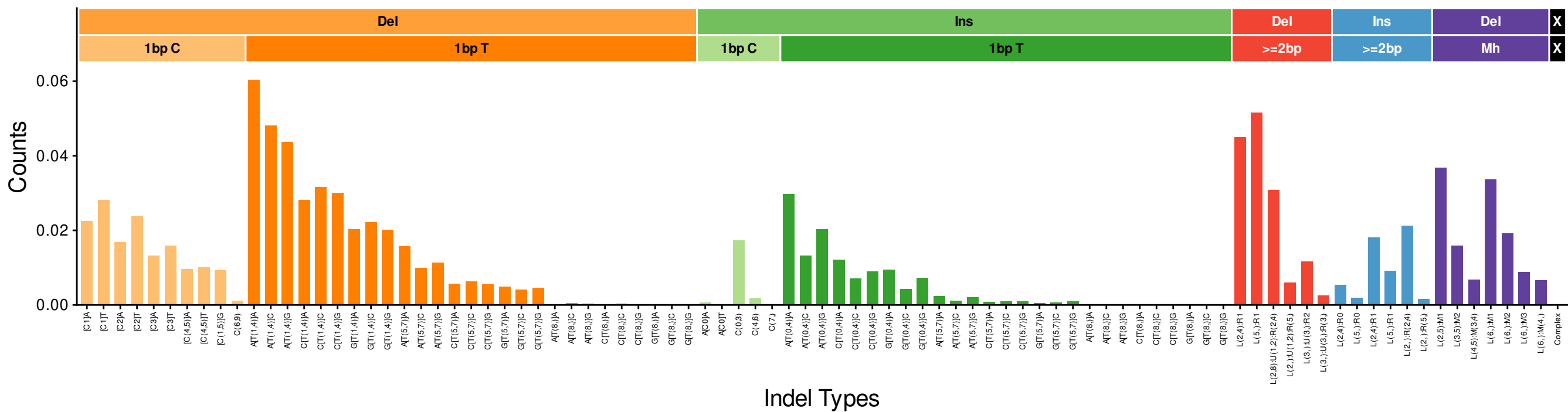
InD29 (cosine: 0.9359)
