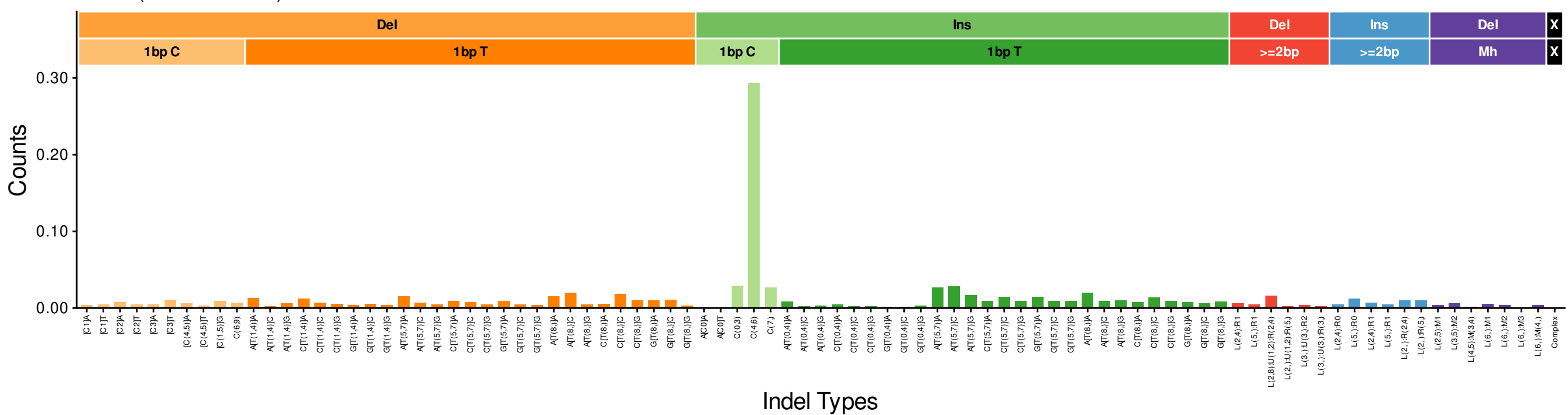
InD30 (euclidean: 0.2512)
