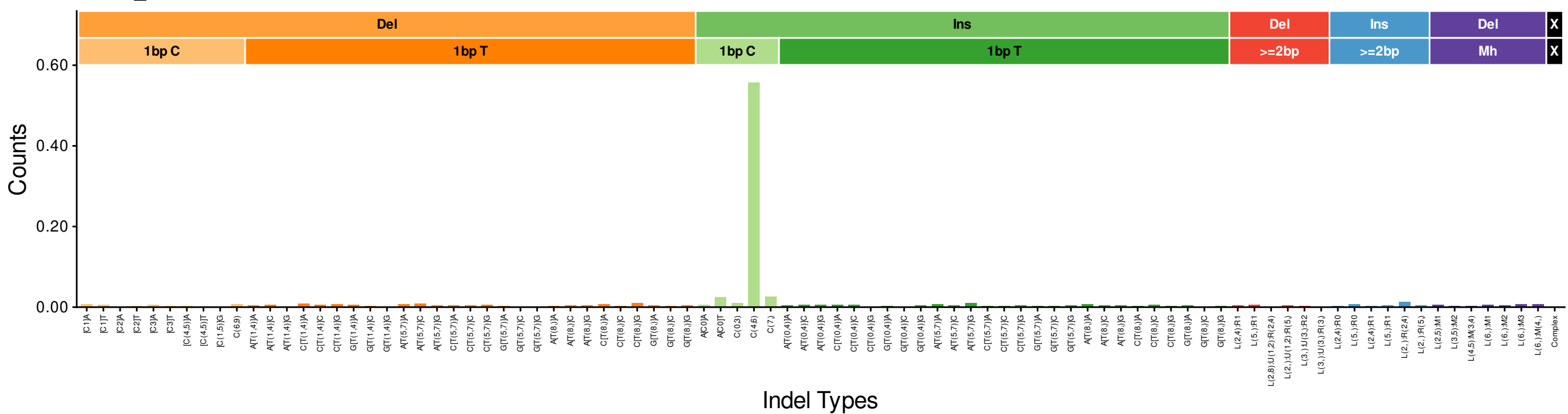
InD26 (cosine: 0.9692)
