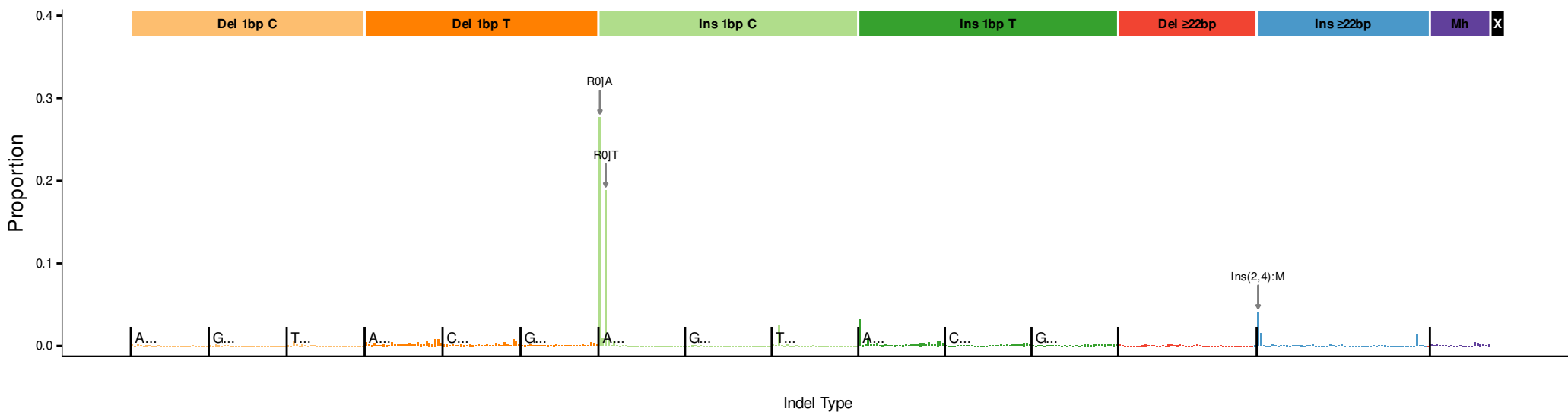
InsDel_D
