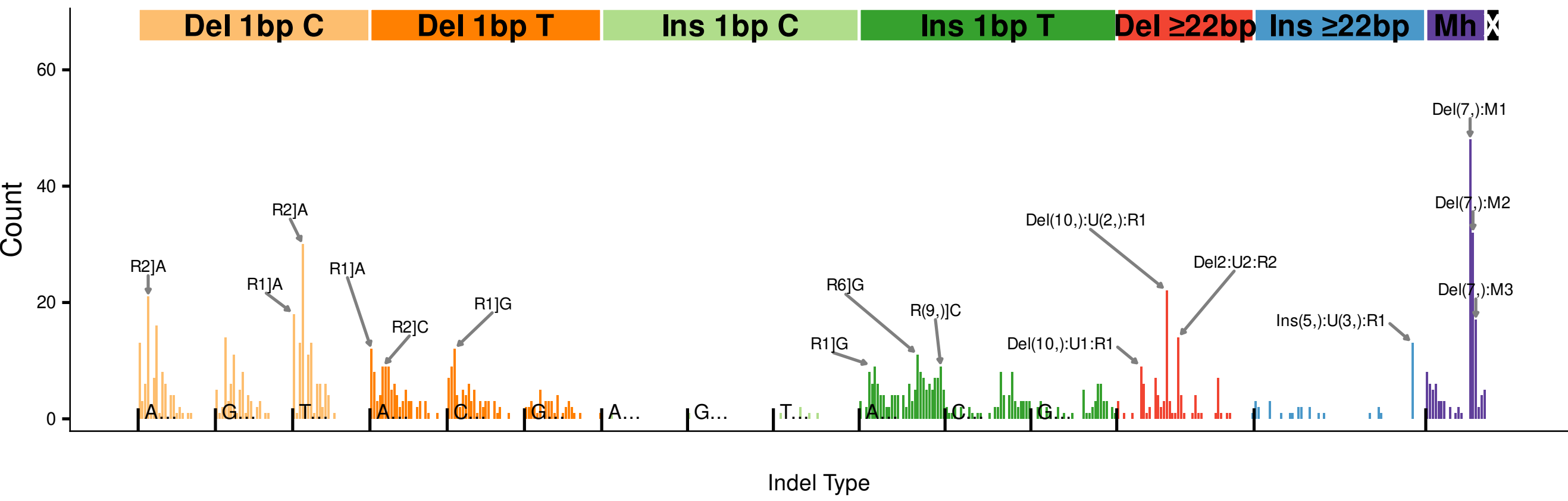
Liver..SP112290 (cosine: 0.9522)
