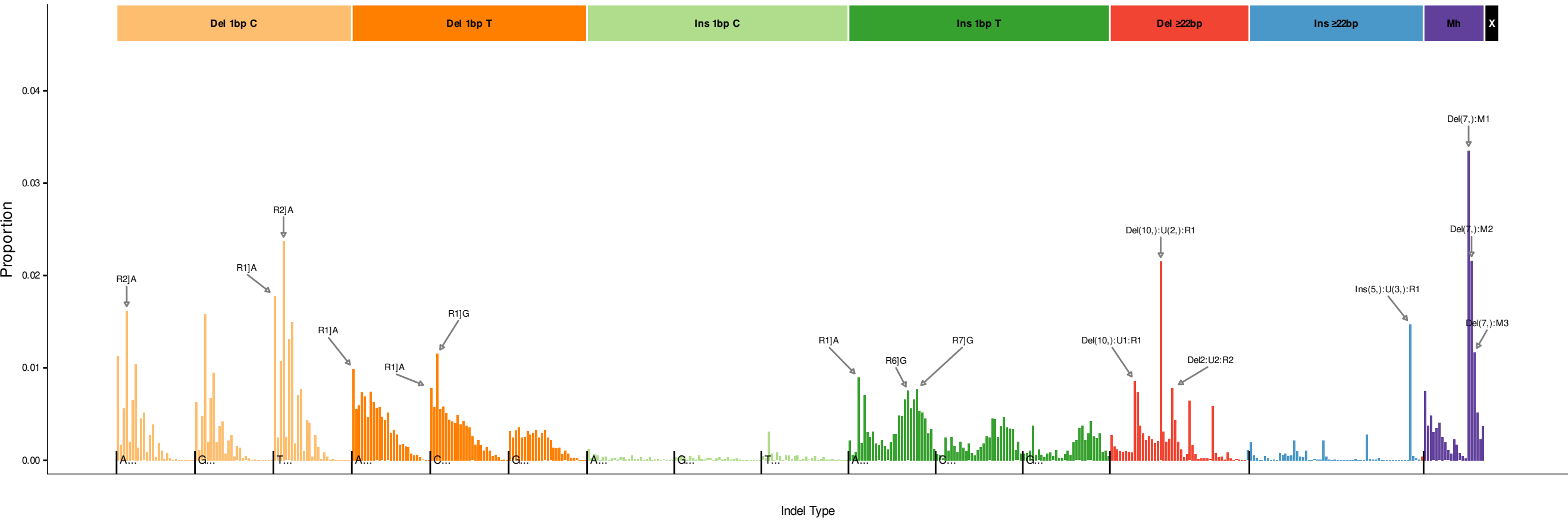
InsDel5b
