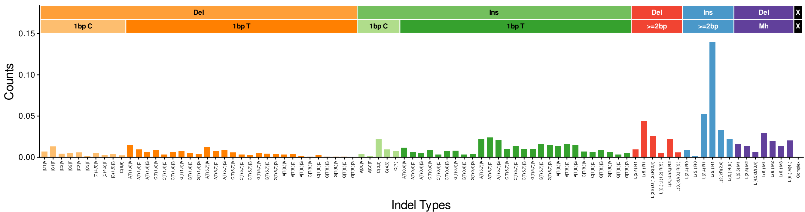
InD23 (cosine: 0.8612)
