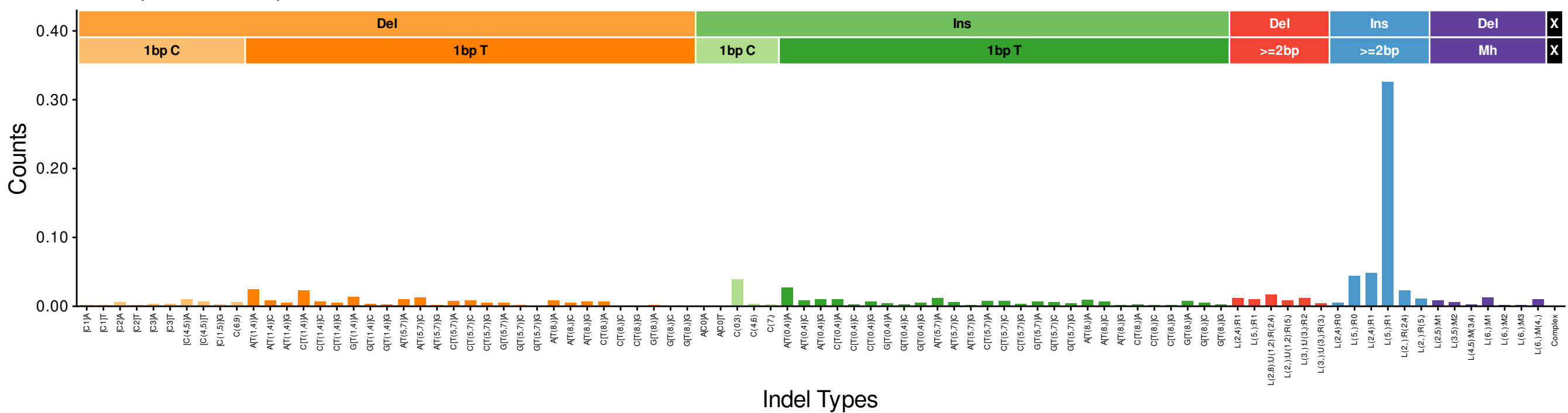
InD29 (euclidean: 0.1702)
