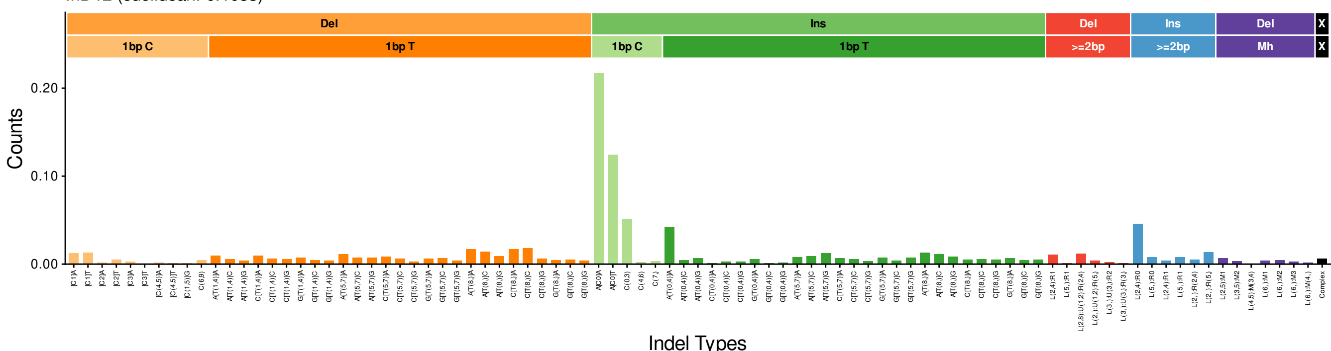
InD12 (euclidean: 0.1033)
