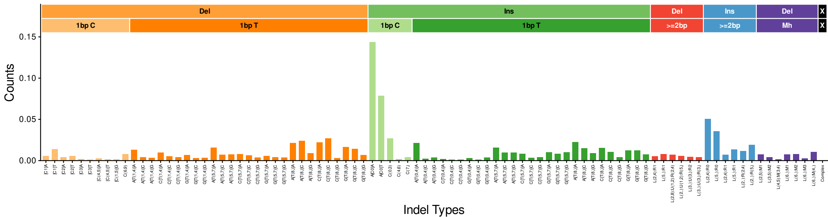
InsDel_D
