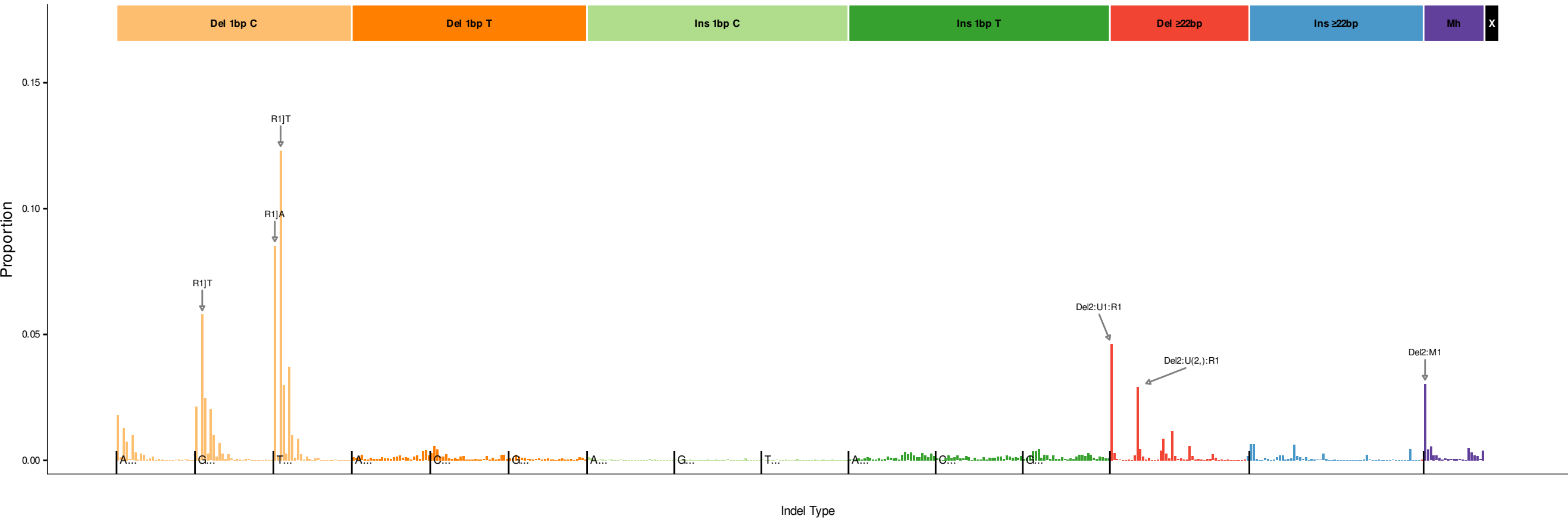
InsDel_A_alpha
