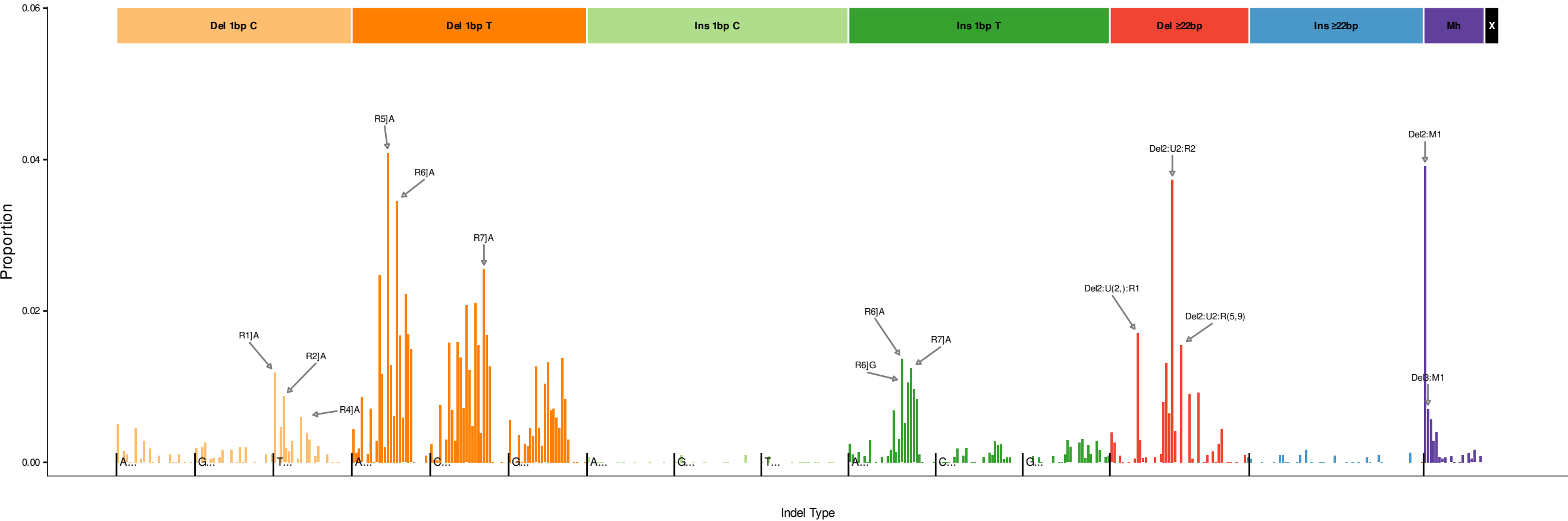
InsDel_K_alpha
