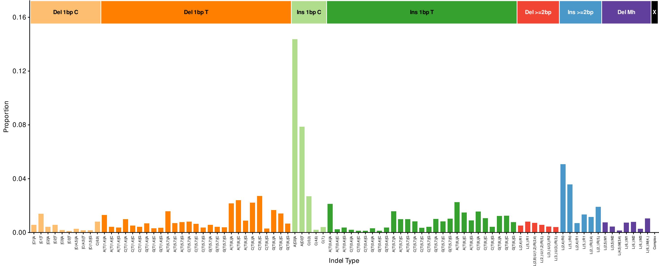
Colon..CPCT02040258T (cosine: 0.9753)
