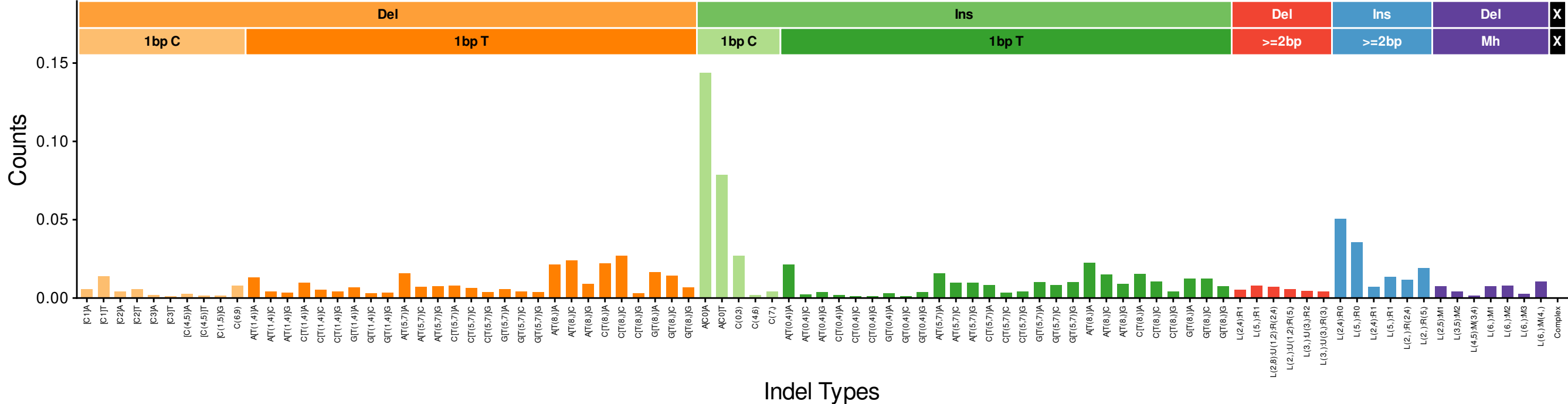
InsDel_D (euclidean: 0.1033)
