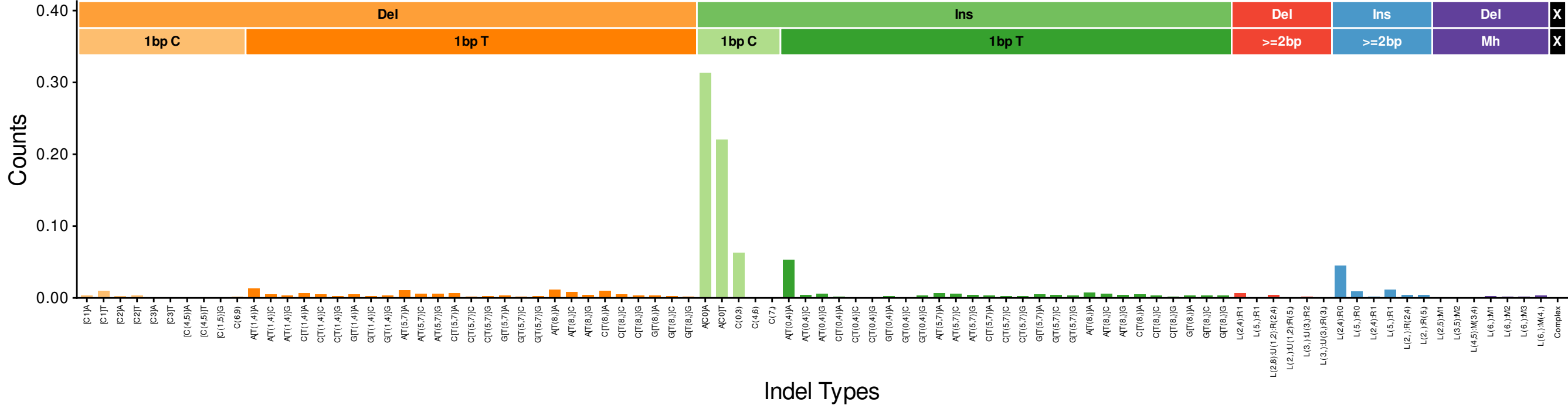
InsDel_D (euclidean: 0.1033)
