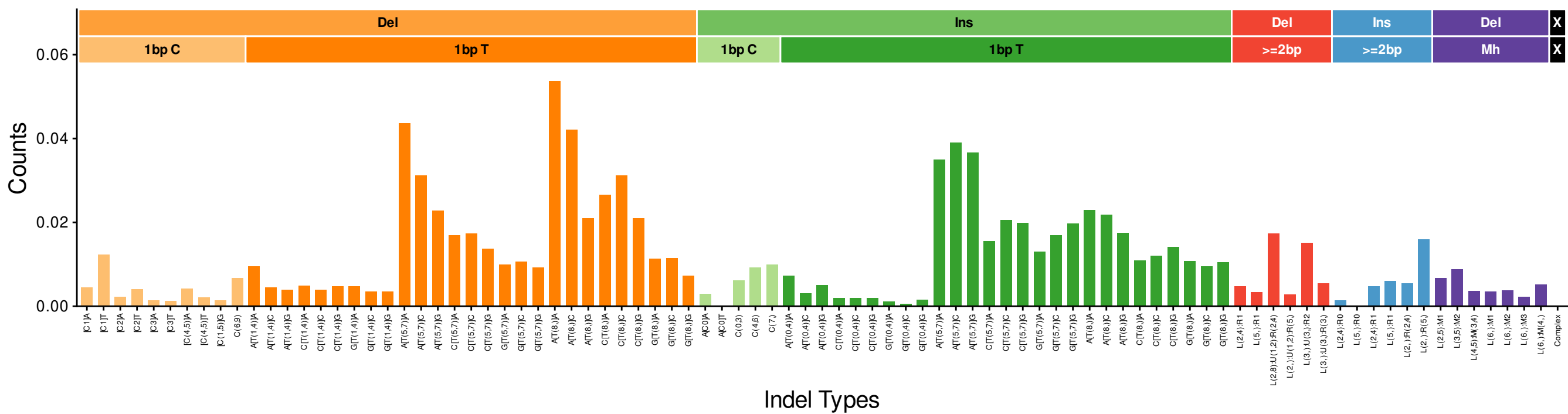
InsDel1d (euclidean: 0.0690)
