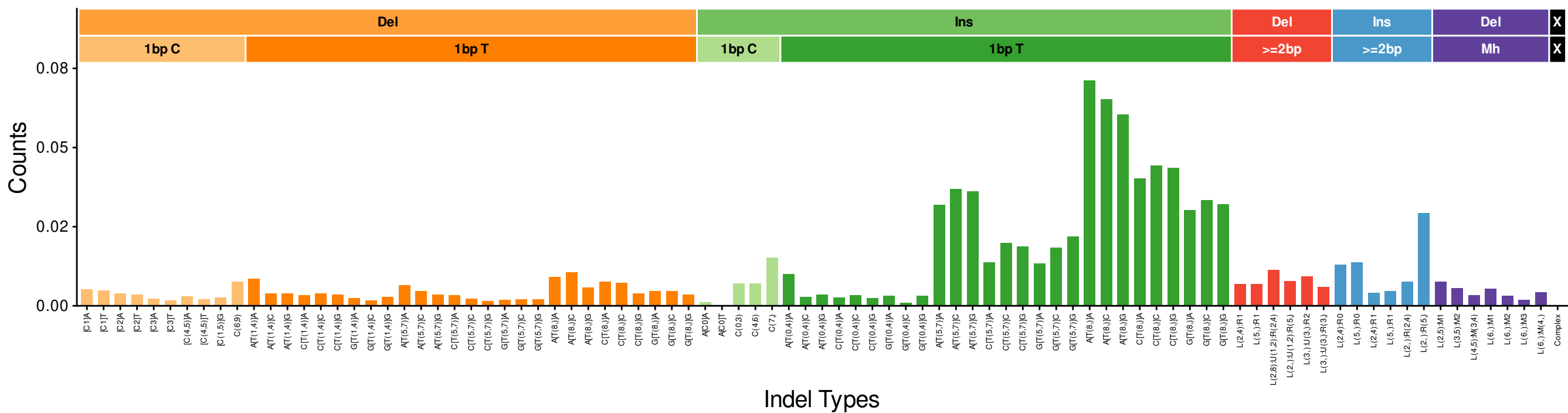
InsDel1a (euclidean: 0.0363)
