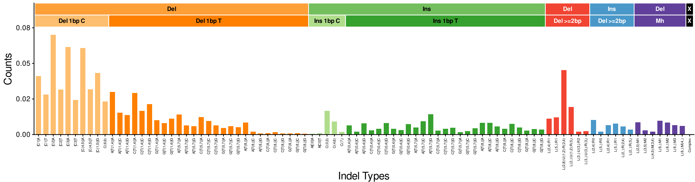
Lung..SP57735 (cosine: 0.9556)
