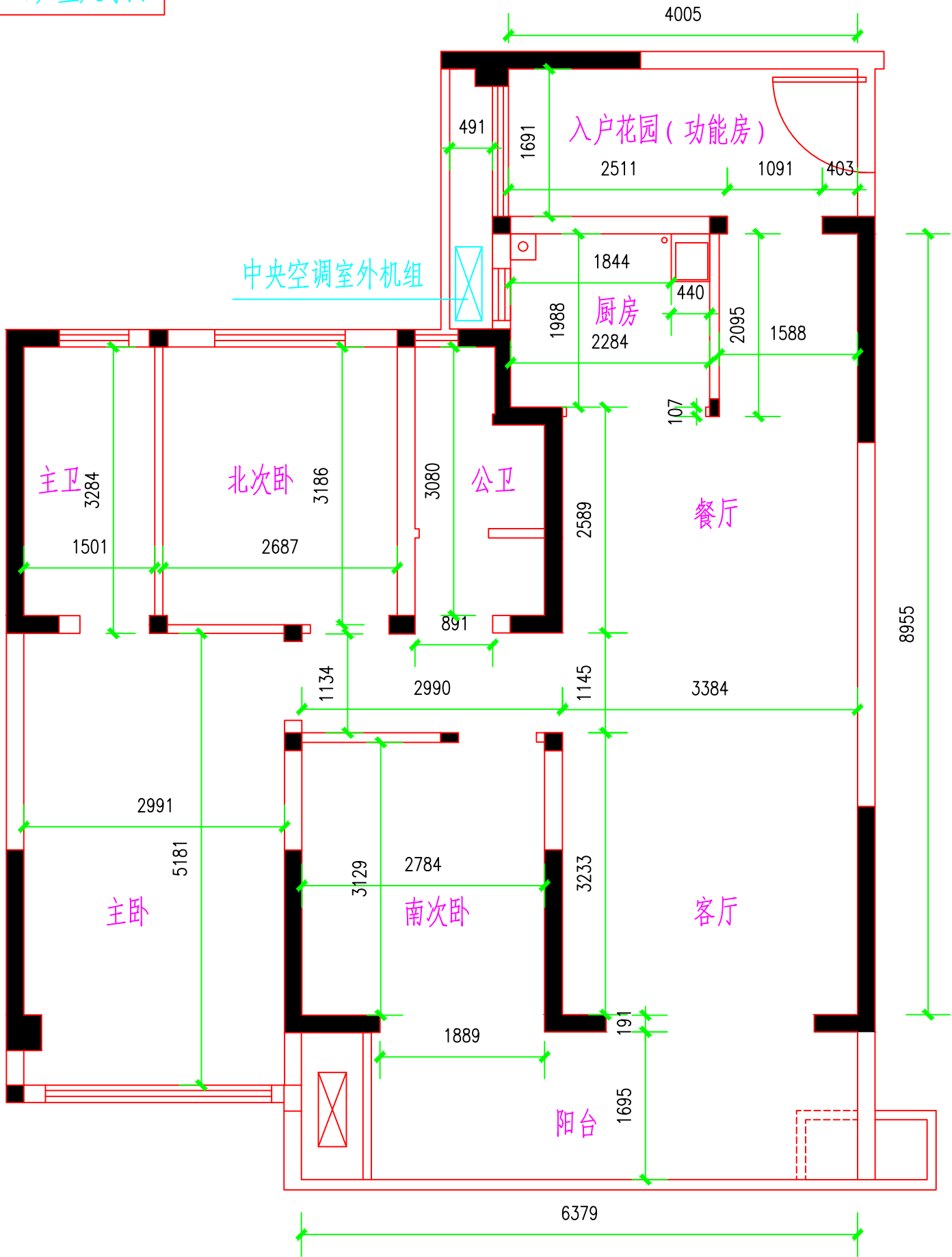
A-1 户型尺寸图
