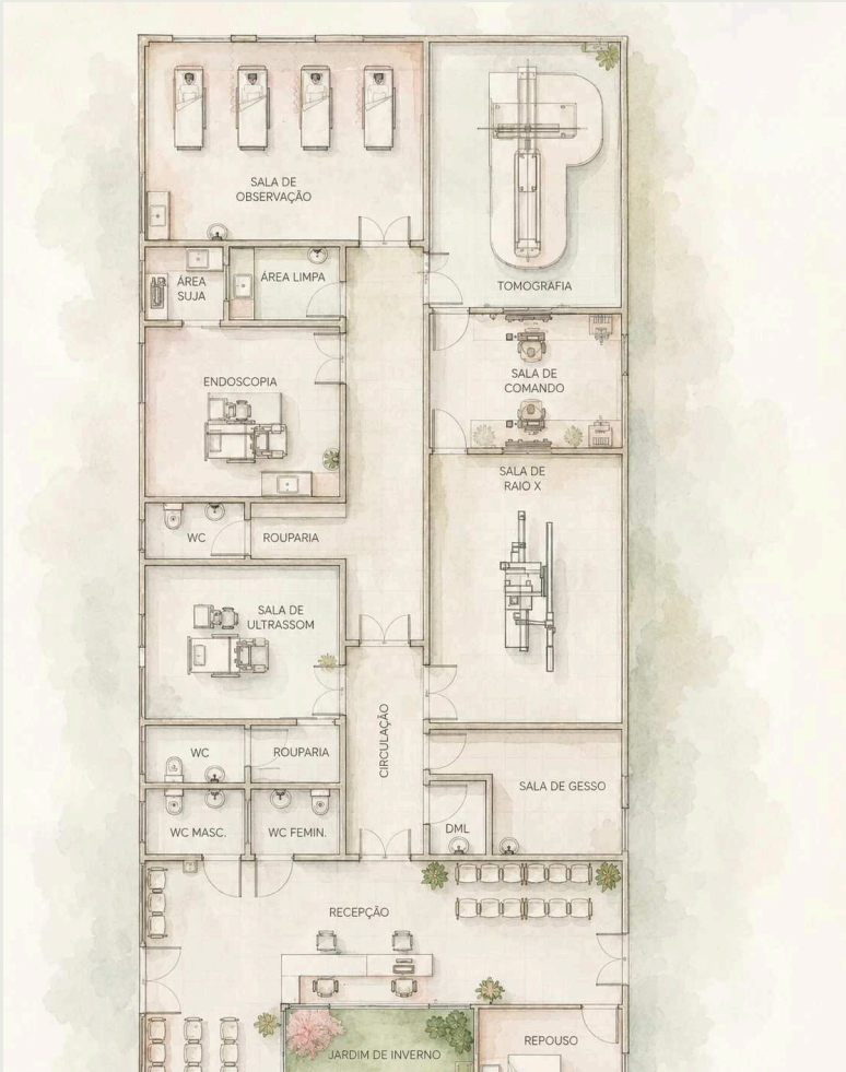
PLANTA DA REFORMA • PROJETO DE AUTORIA PRÓPRIA
