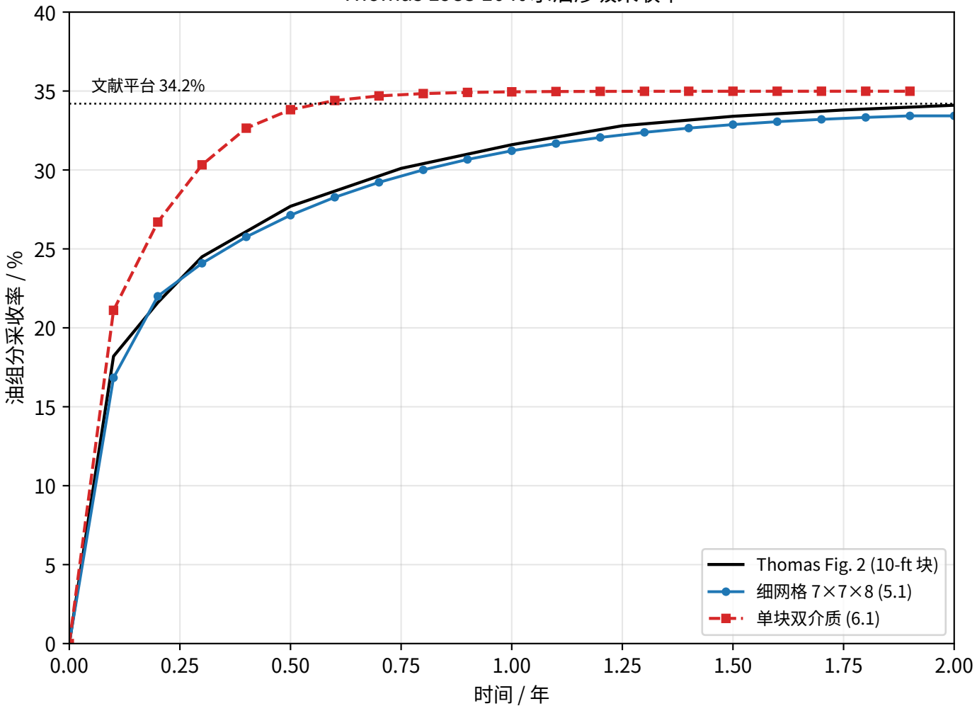
Thomas 1983 10 ft 水油渗吸采收率
