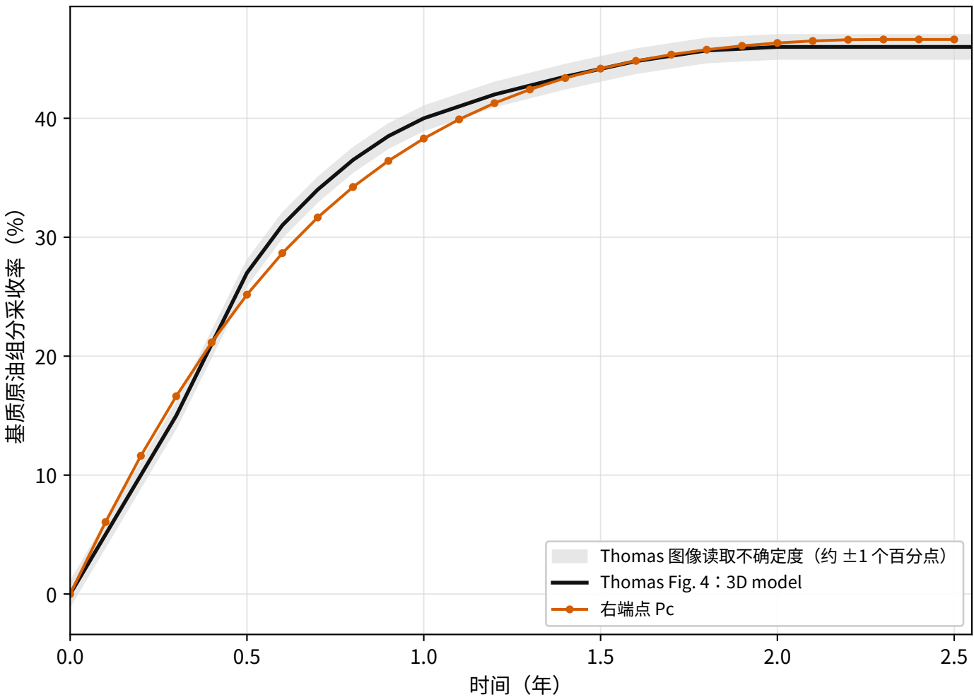
Thomas 10 ft 细网格：PVT 动态静水裂缝压力
