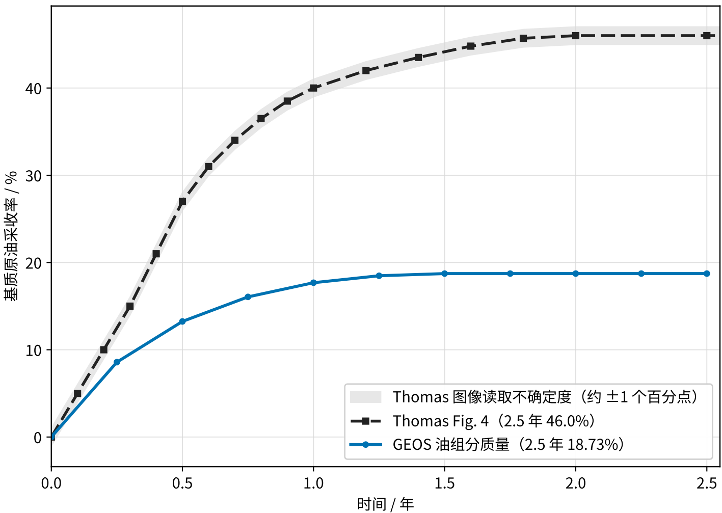
Thomas 10 ft 双重介质单块：气油重力排驱
