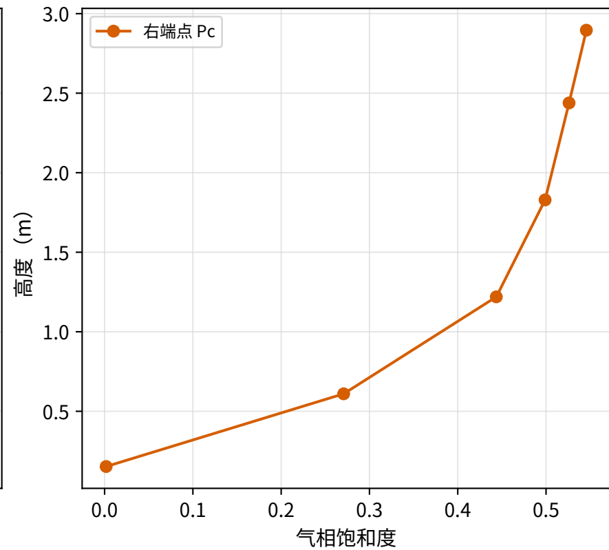
2.5 年基质气相饱和度
