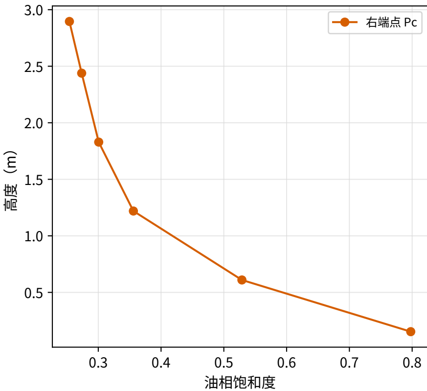
2.5 年基质油相饱和度
