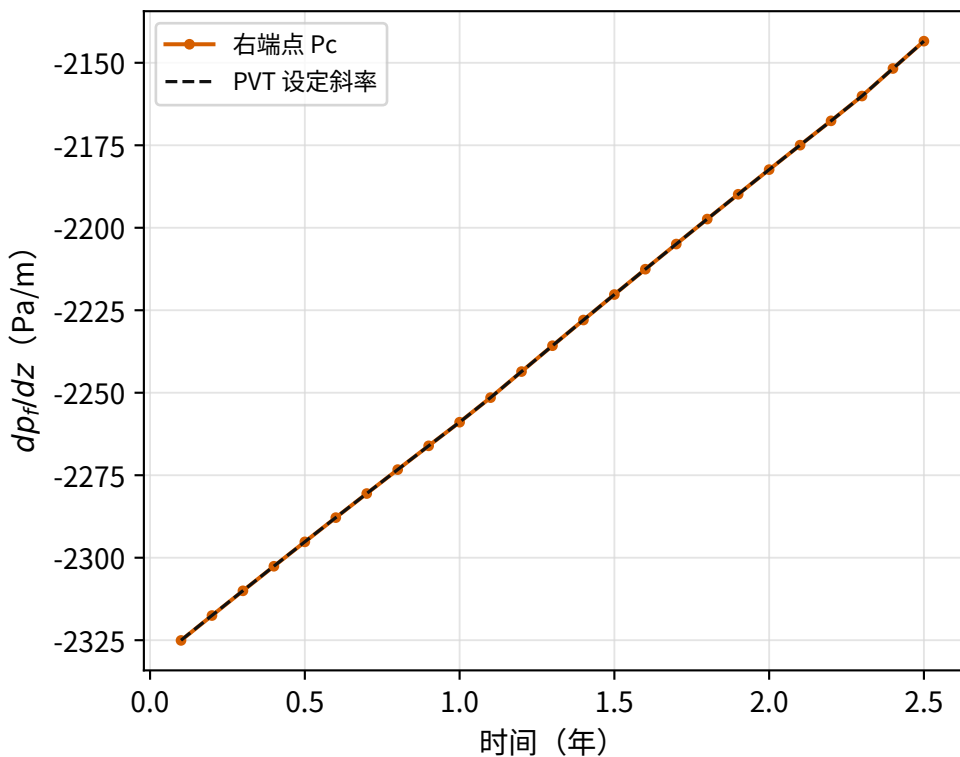
裂缝气体静水压力梯度
