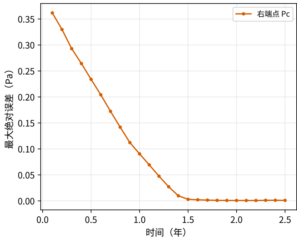
裂缝压力对设定函数的误差
