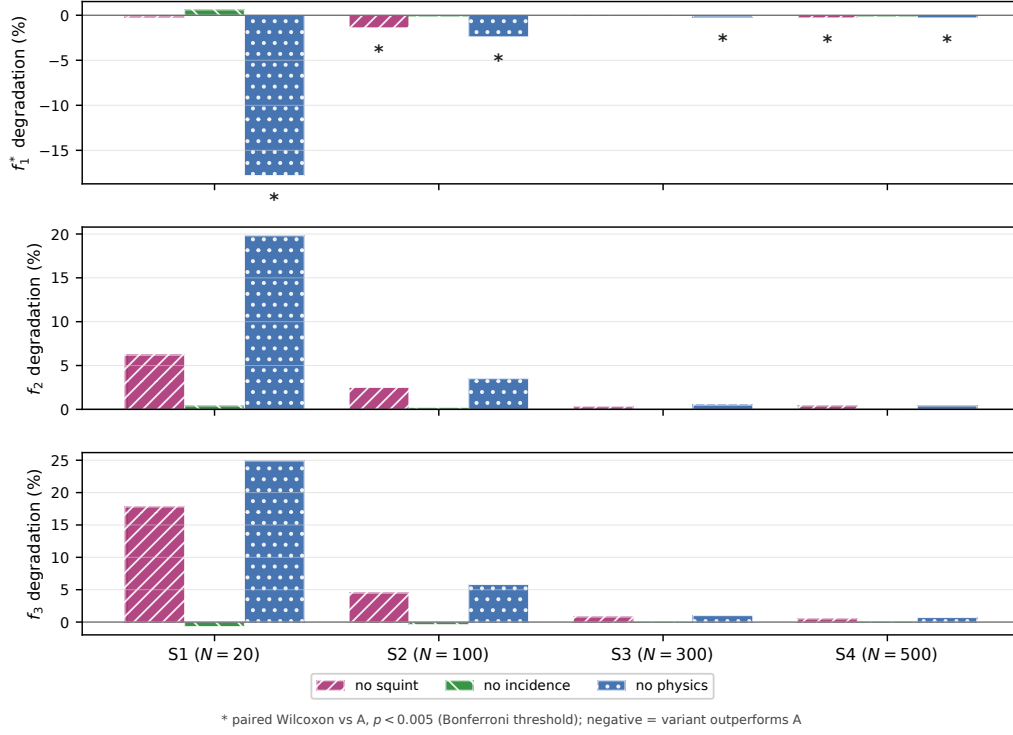
Figure 5: 四种目标函数变体 (B–D) 与四类场景 (S1–S4) 下的消融结果。柱状图表示相对完整物理基线 A 的归一化收益 f_1^* 与事后几何质量指标 f_2 、 f_3 的退化 (负值表示变体优于 A)；星号标记与 A 配对 Wilcoxon 比较达到 Bonferroni 阈值 ( p < 0.05/12 )。
