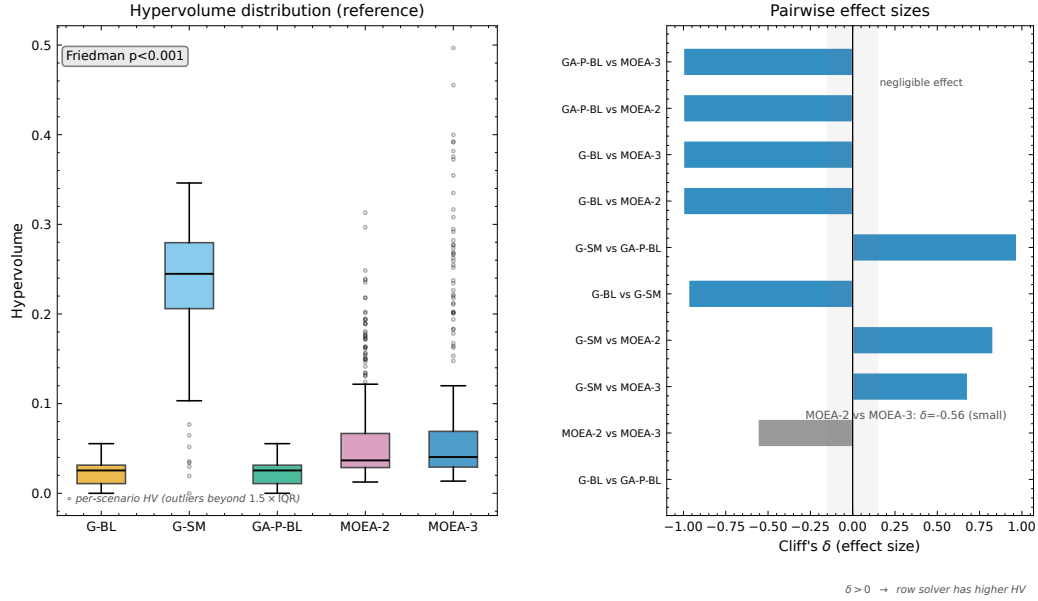
Figure 1: 统计验证：（左）超体积分布；（右）配对效应量，用匹配对符号统计量 \delta_{\text{pairs}} = (W - L)/n （在场景配对下等于 Cliff's \delta ）；灰色波段标记 Romano et al. (2006) 可忽略效应区 ( |\delta| < 0.147 ；仅供参考，配对比较的常规未配对 \delta 更弱)，见 § 5.3。
