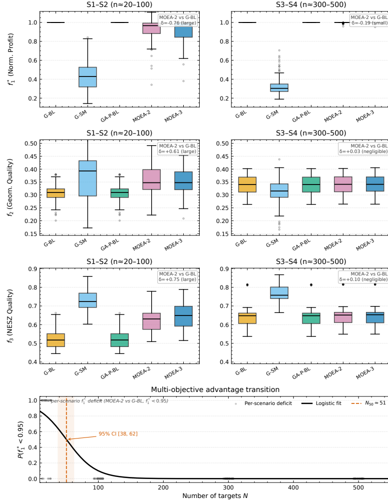
Figure 3: 尺度敏感性：（上）稀疏（S1-S2）与密集（S3-S4）场景类别下归一化收益 f_1^* 、几何质量 f_2 与辐射质量 f_3 的逐目标分布；（下）覆盖率差距比例（ f_1^* < 0.95 ）的逻辑回归拟合，附逐场景抖动指示点。
