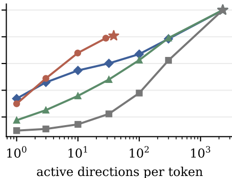
Gemma 2 2B
